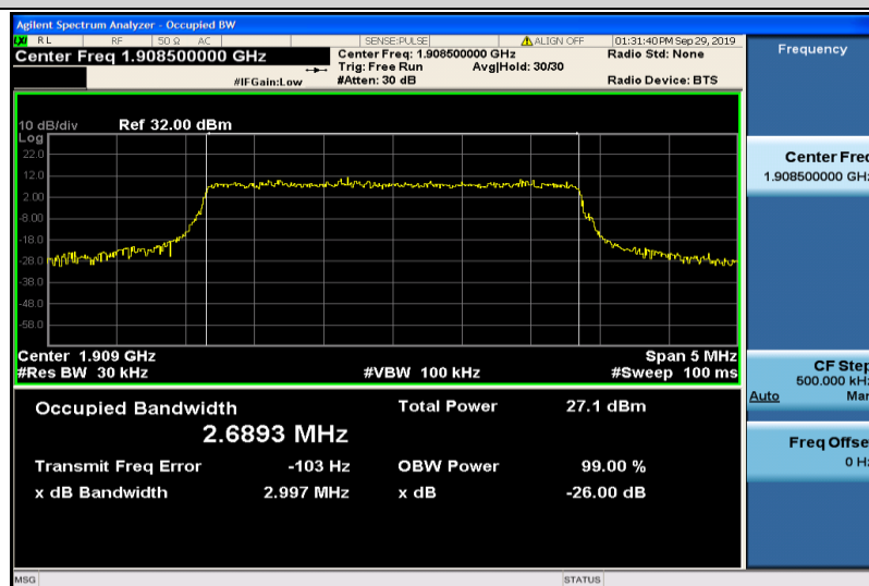
Band2-3MHz-QPSK-19185-15RB#0-2.6893
