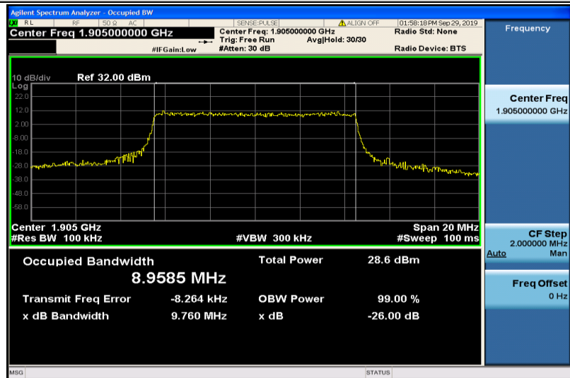
Band2-10MHz-QPSK-19150-50RB#0-8.9585
