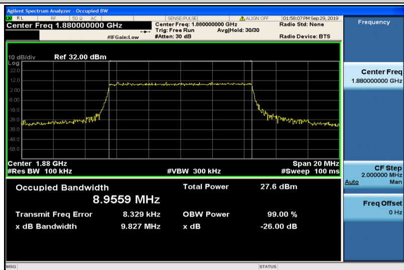
Band2-10MHz-16QAM-18900-50RB#0-8.9559
