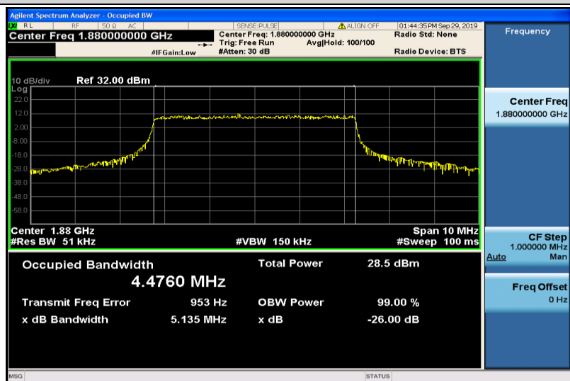
Band2-5MHz-QPSK-18900-25RB#0-4.4760
