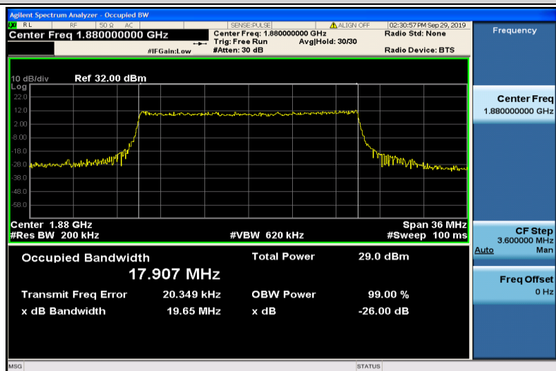
Band2-20MHz-QPSK-18900-100RB#0-17.907
