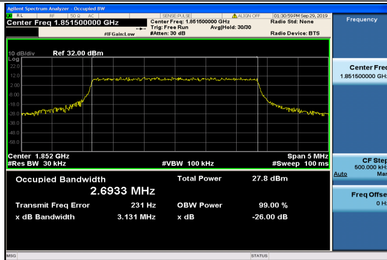
Band2-3MHz-QPSK-18615-15RB#0-2.6933
