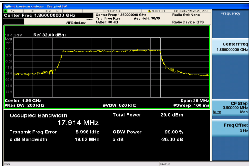
Band2-20MHz-QPSK-18700-100RB#0-17.914
