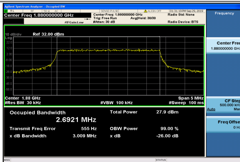
Band2-3MHz-QPSK-18900-15RB#0-2.6921
