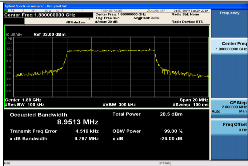
Band2-10MHz-QPSK-18900-50RB#0-8.9513
