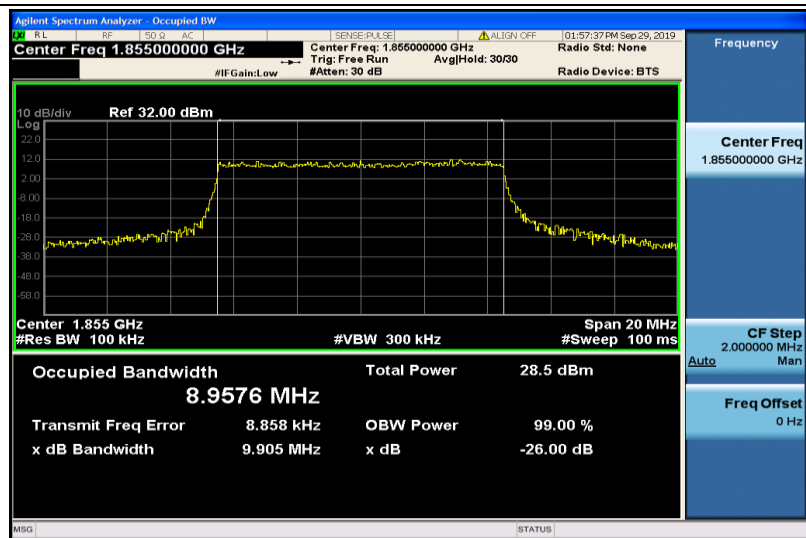
Band2-10MHz-QPSK-18650-50RB#0-8.9576
