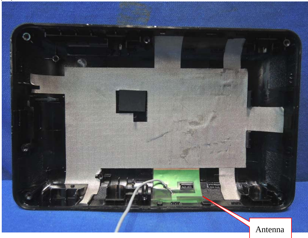
(12) EUT Photo
