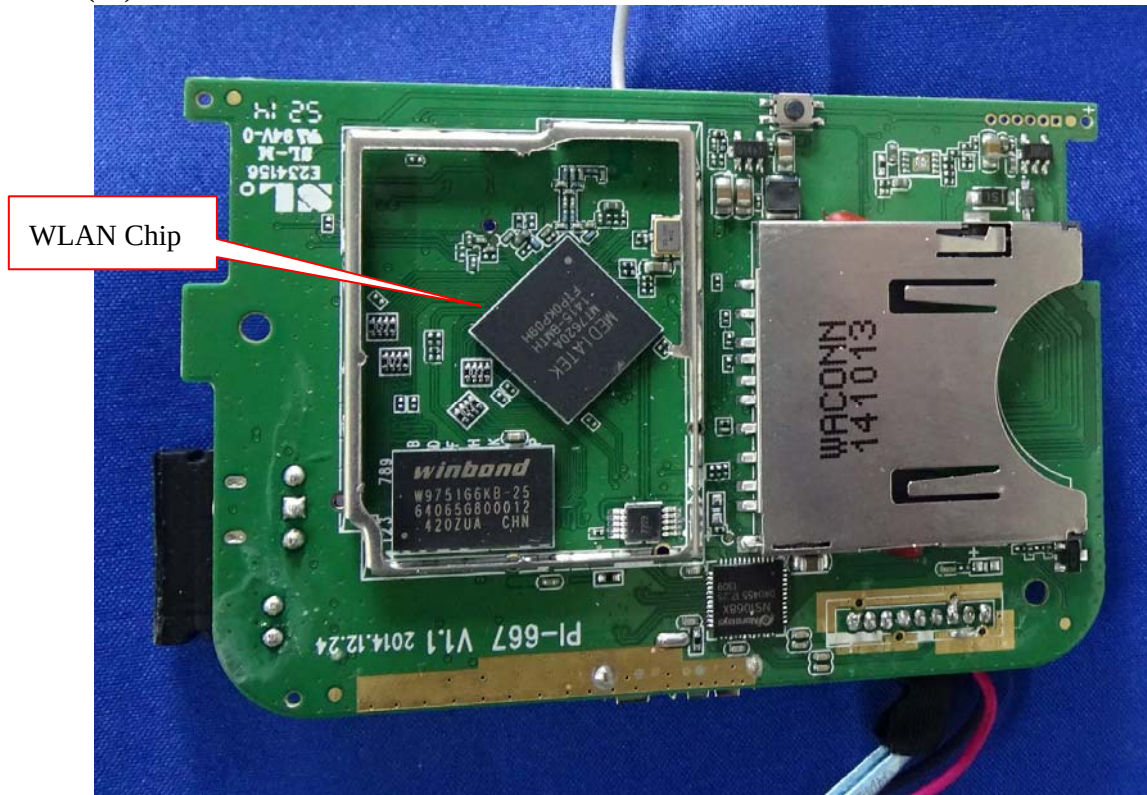
(16) EUT Photo
