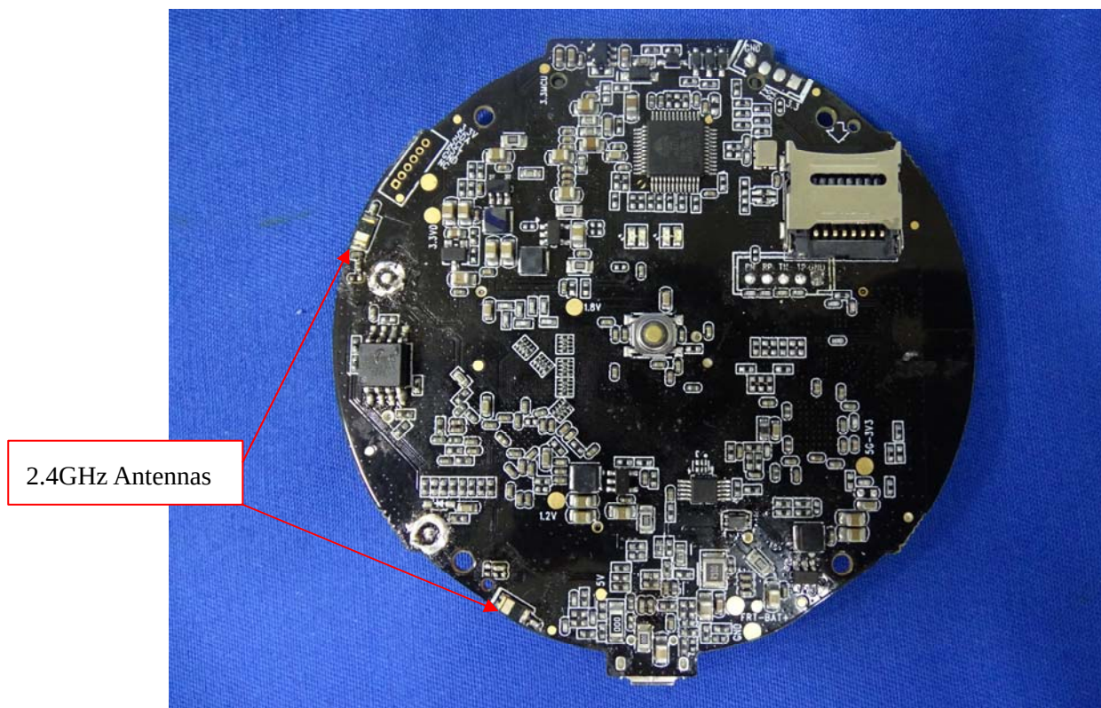
(13) EUT Photo
