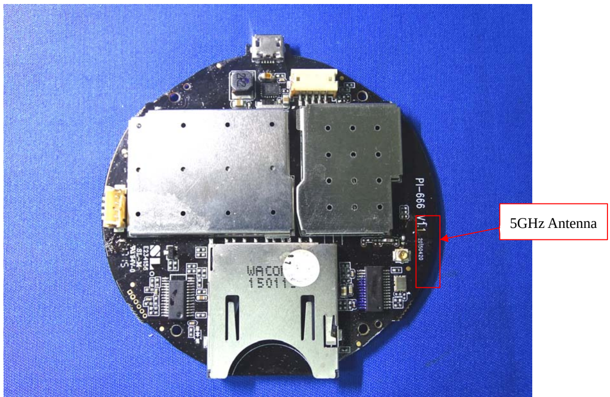
(18) EUT Photo
