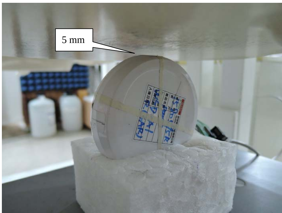
EUT Top
