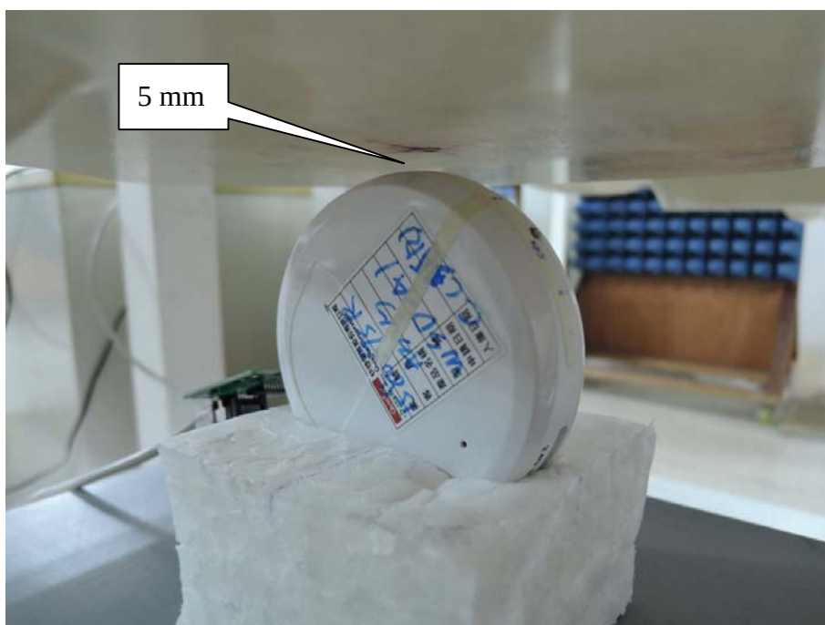
EUT Left-Side 1
