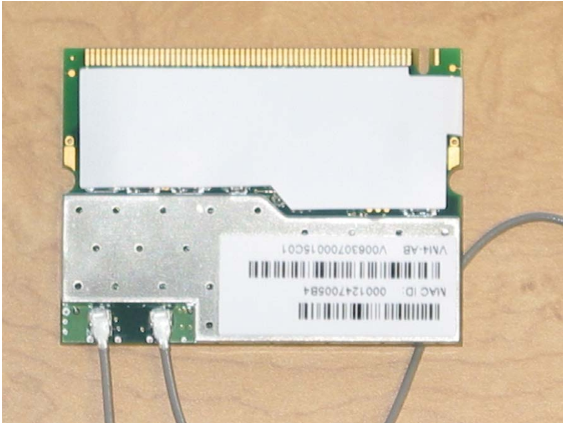
Mini PCI module front
