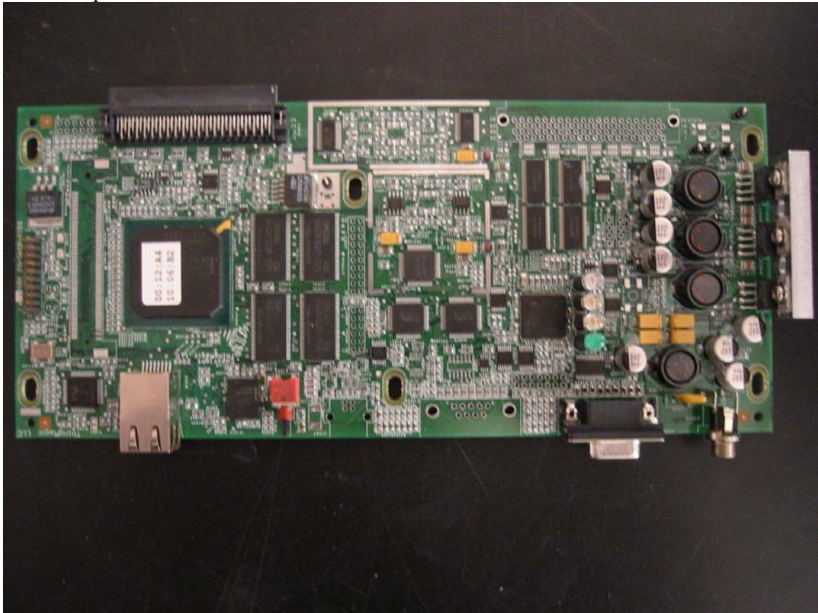
PCB 2 Top
