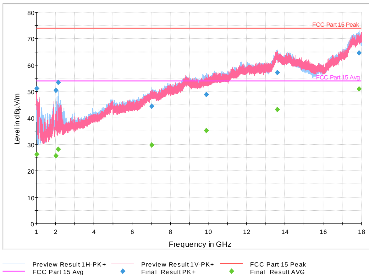
Figure 30. 1-18GHz, 902.75 MHz
