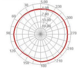
2400.000MHz H
