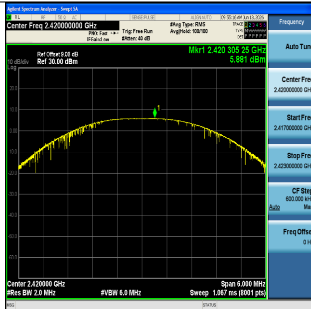
SRD-Ant1-2420-PASS
