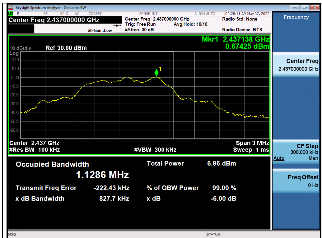
Test_Graph_GFSK_ANT1_2437_DTSBW
