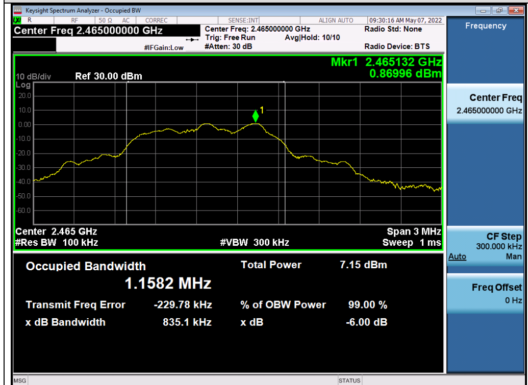
Test_Graph_GFSK_ANT1_2465_DTSBW
