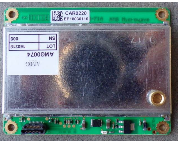
MW radar antenna & Module
