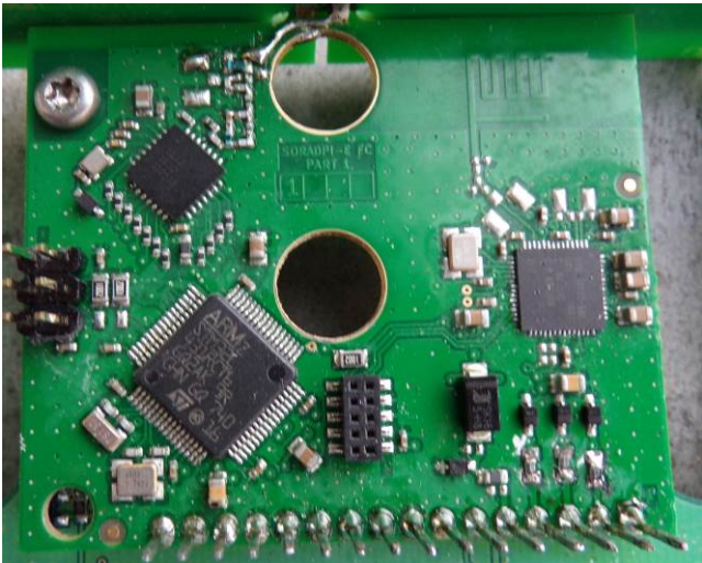
BLE board
