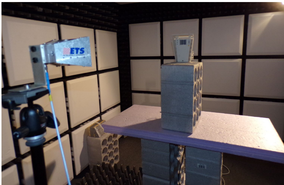
FAC setup (18GHz-25GHz / 1m)
