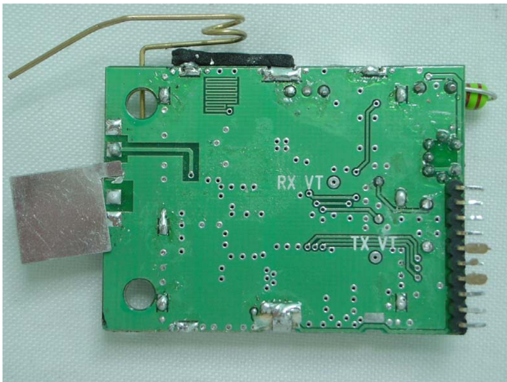
RF Module Rear
