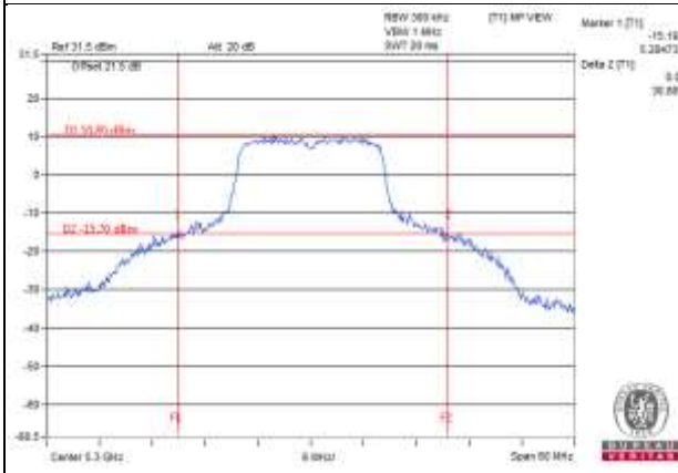
802.11a – CH60
