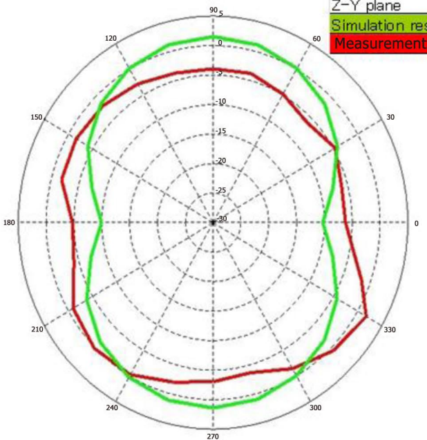
2480MHz
