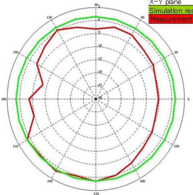
2480MHz
