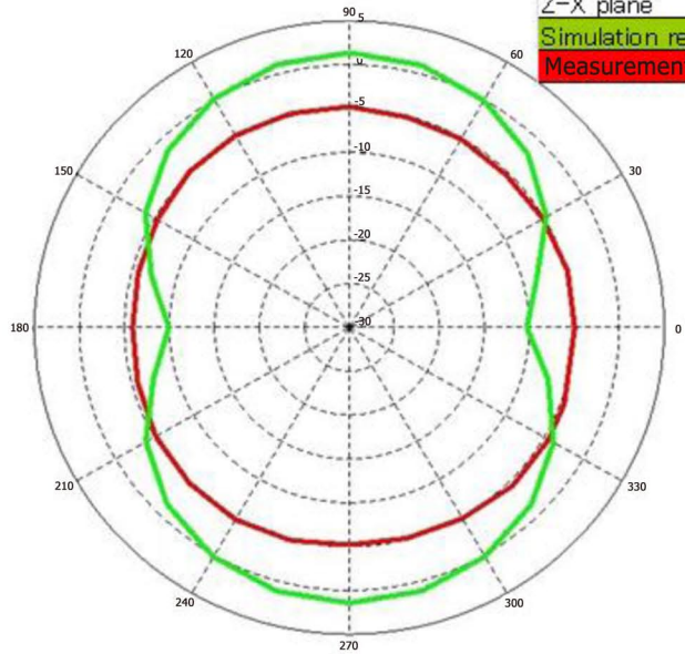
2480MHz
