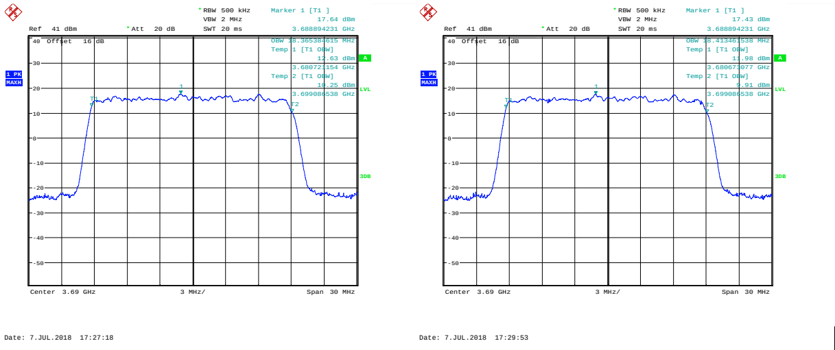
99 % Bandwidth; QPSK; 3690 MHz; MIMO A.
