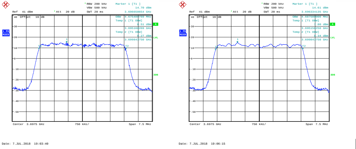
99 % Bandwidth QPSK; 3697.5 MHz; MIMO A.
