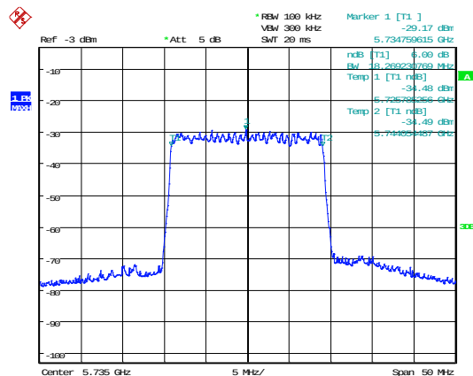
QPSK 5735 MHz
