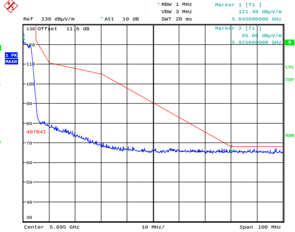
256QAM
