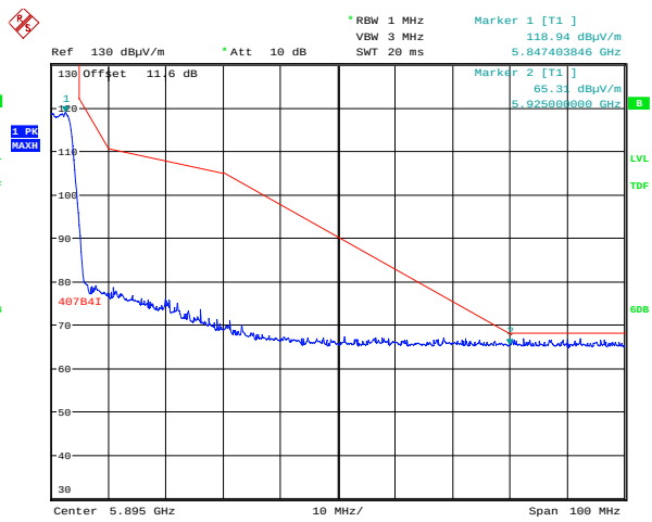
QPSK
