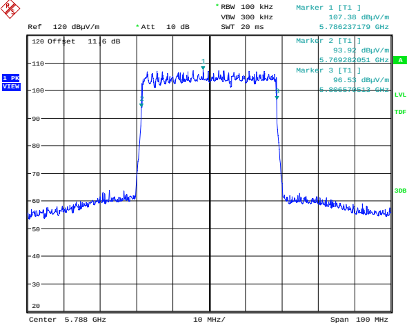
QPSK 5788 MHz
