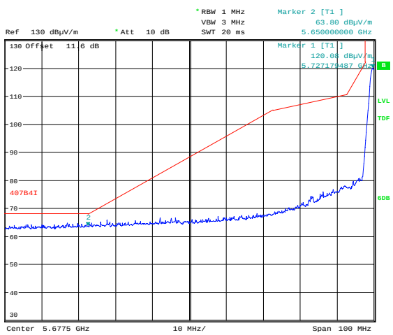
MIMO B
