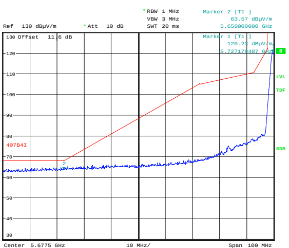
MIMO B
