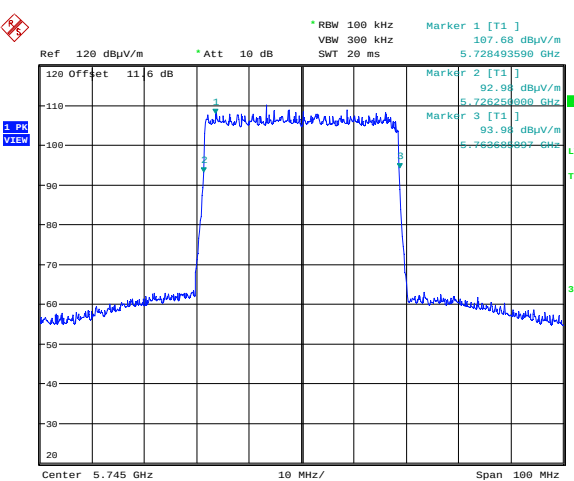
QPSK 5745 MHz
