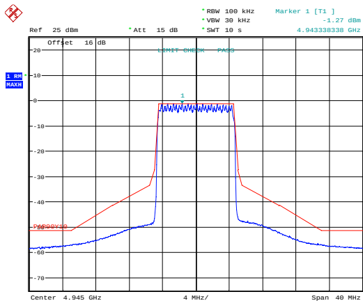
Emission Mask QPSK; MIMO A; 4945 MHz.
