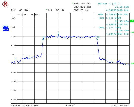
99 % Bandwidth QPSK; 4942.5 MHz; MIMO B.
