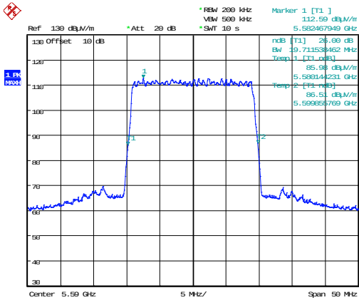
MIMO A
