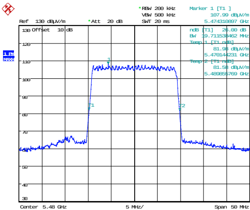
MIMO A
