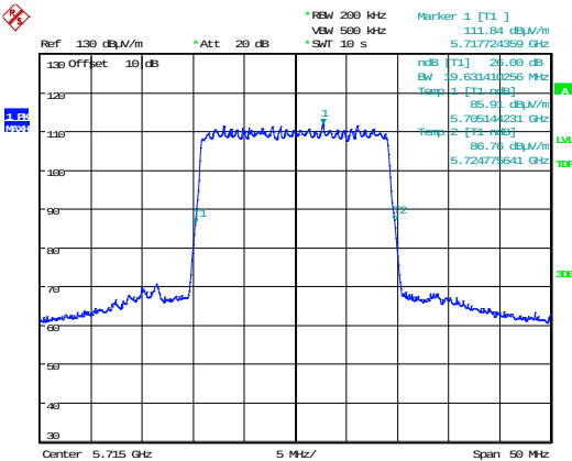
QPSK 5715 MHz
