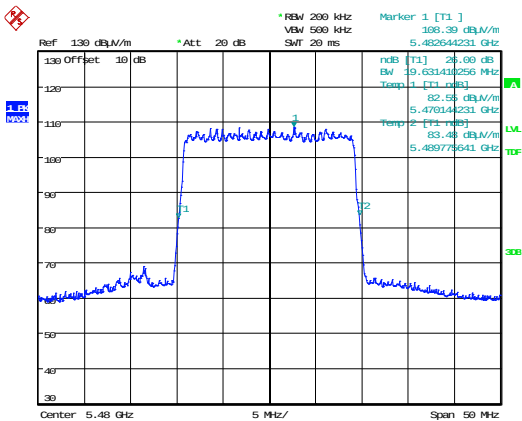
QPSK 5480 MHz
