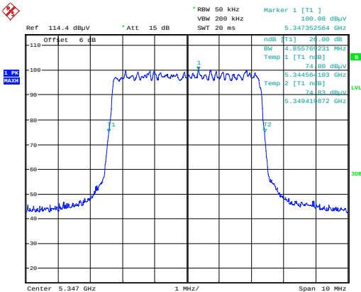
QPSK 5347 MHz
