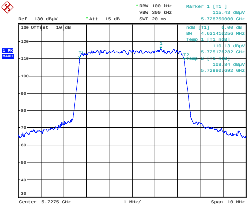
QPSK 5727.5 MHz
