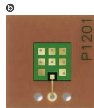
実装特性評価用基板 (CABPB1240用: 40×40mm)
