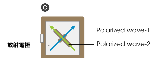
実装特性評価用基板 (CABPB1240用: 40×40mm)
