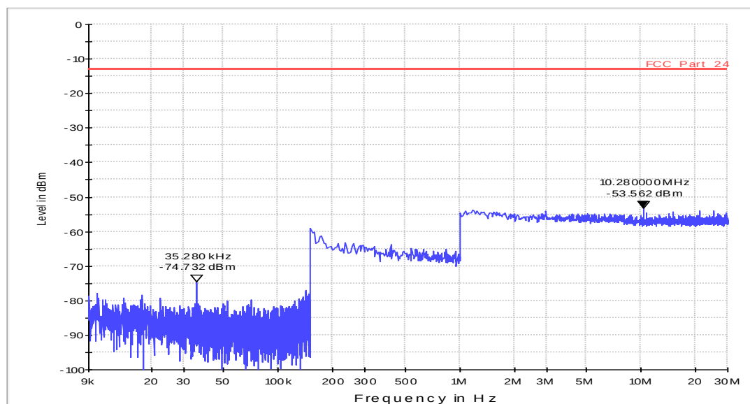
Fula2_FCC_24_Scan1_9kHz_30MHz
