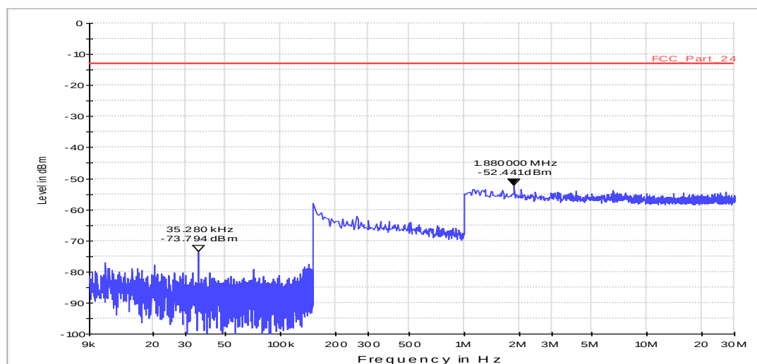
Fula2_FCC_24_Scan1_9kHz_30MHz
