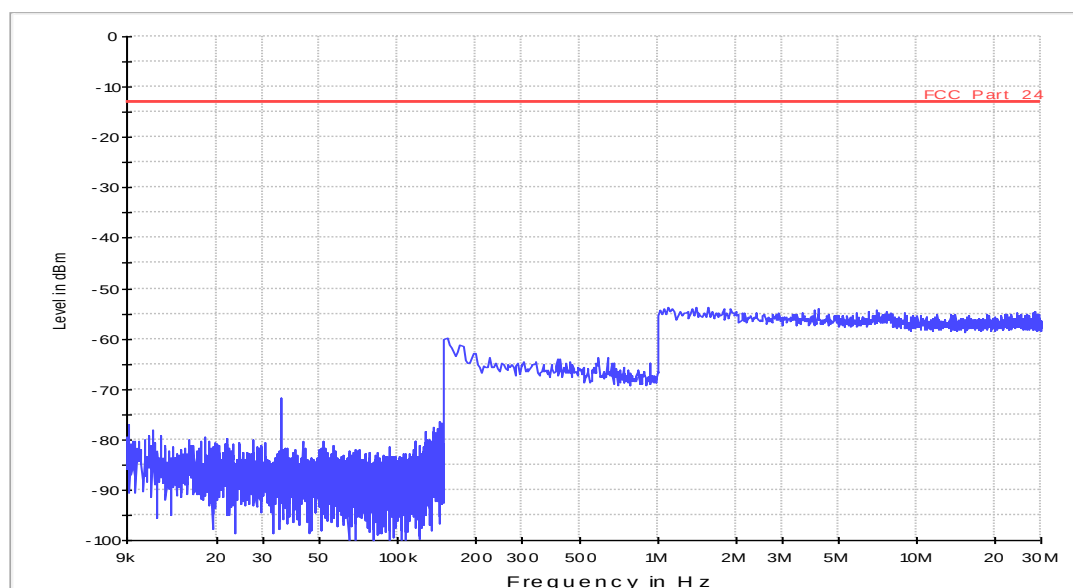
Fula2_FCC_24_Scan1_9kHz_30MHz
