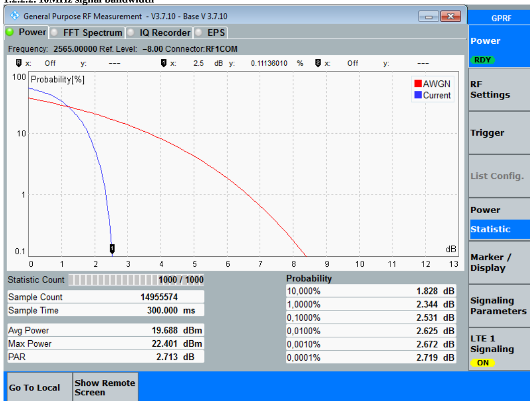
Diagram: Ch21400_QPSK_50RB_10MHz
