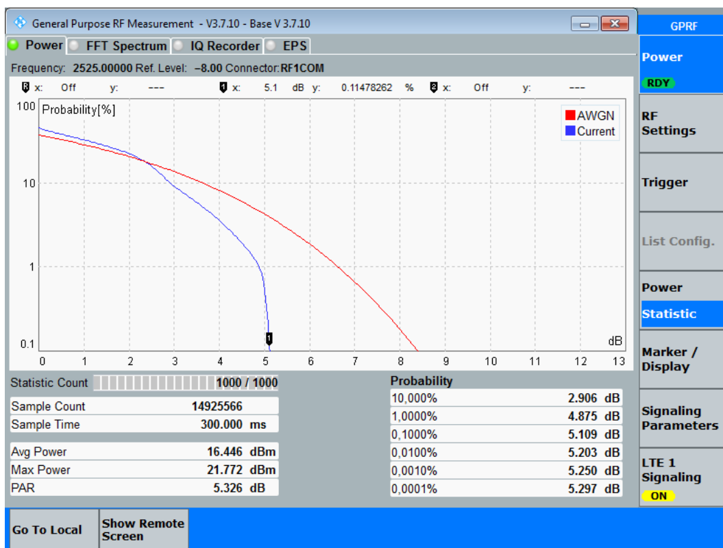
Diagram: Ch21000_QAM_1RB_low_10MHz
