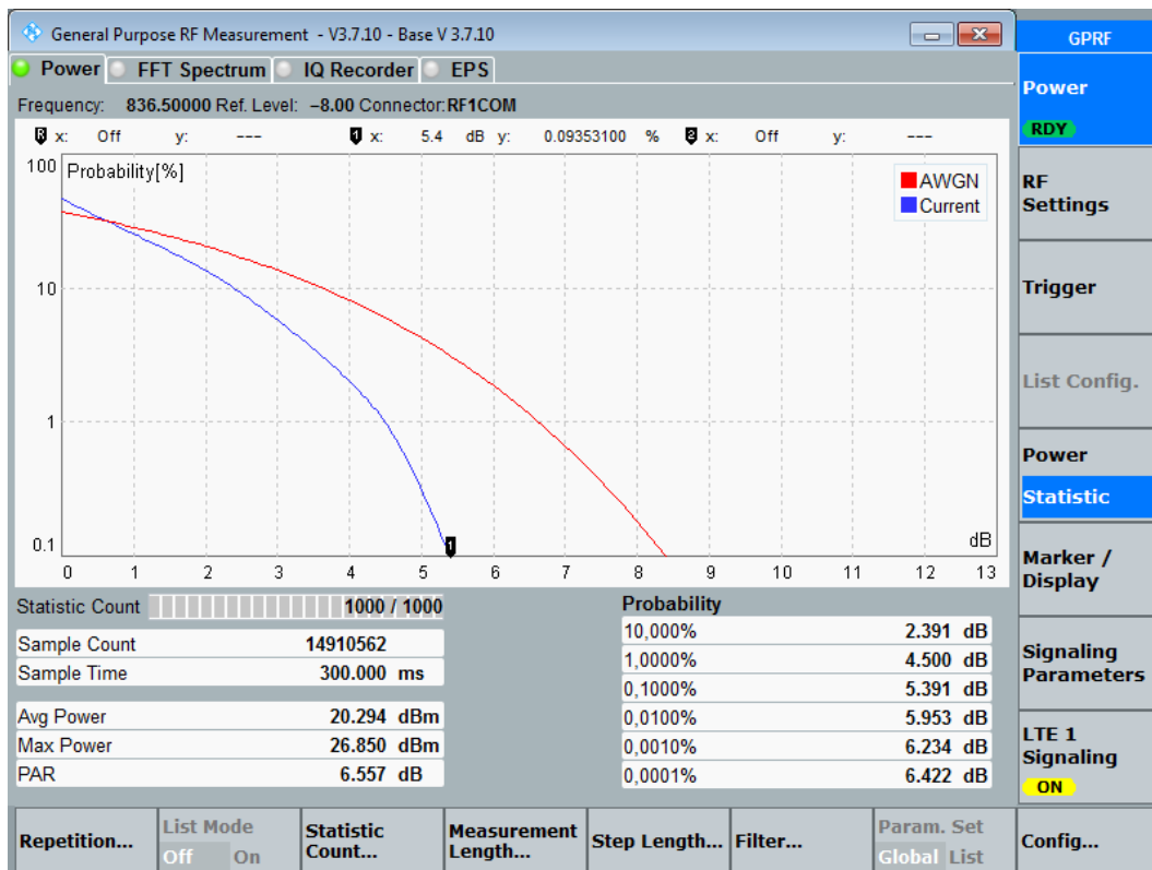
Diagram: Ch20525_QPSK_25RB_5MHz
