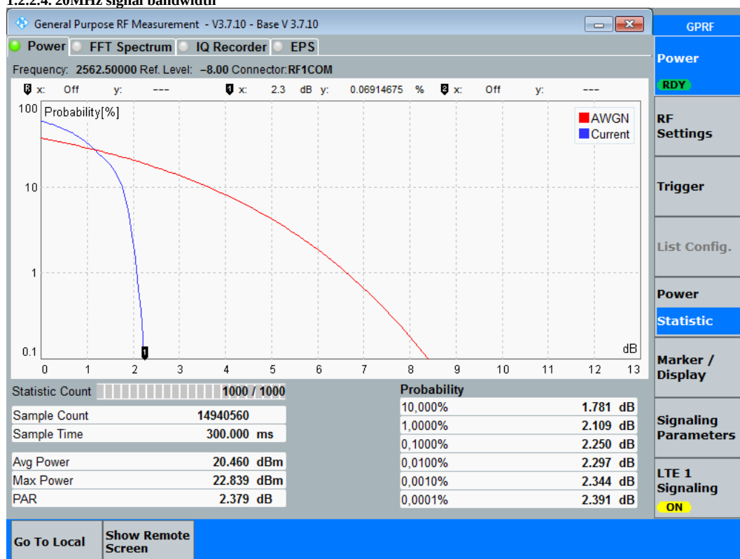
Diagram: Ch21375_QPSK_75RB_20MHz
