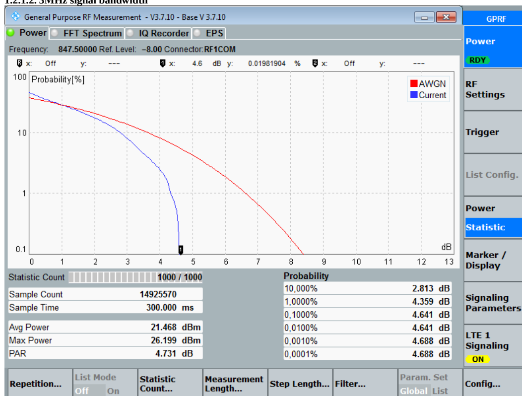
Diagram: Ch20635_QPSK_1RB_low_3MHz
