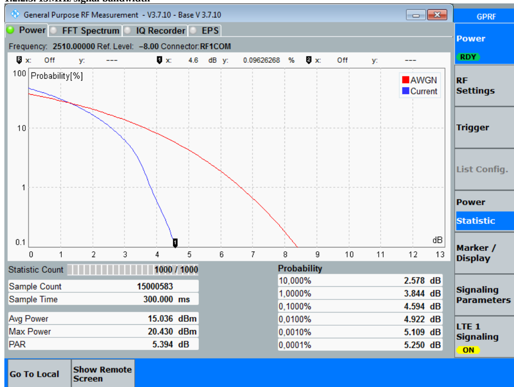
Diagram: Ch20850_QPSK_25RB_15MHz
