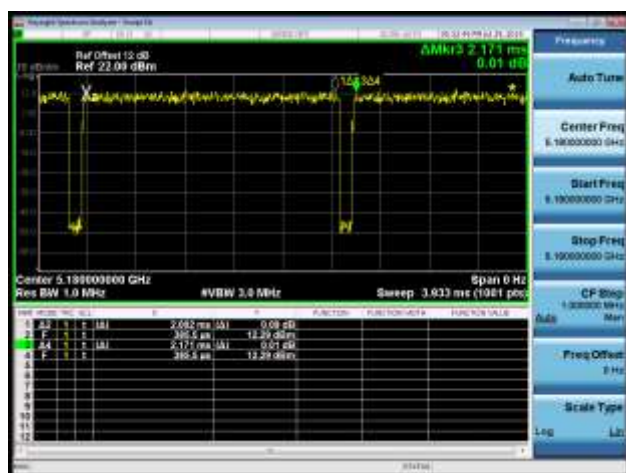
802.11a
