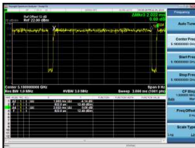
802.11n(20MHz)
