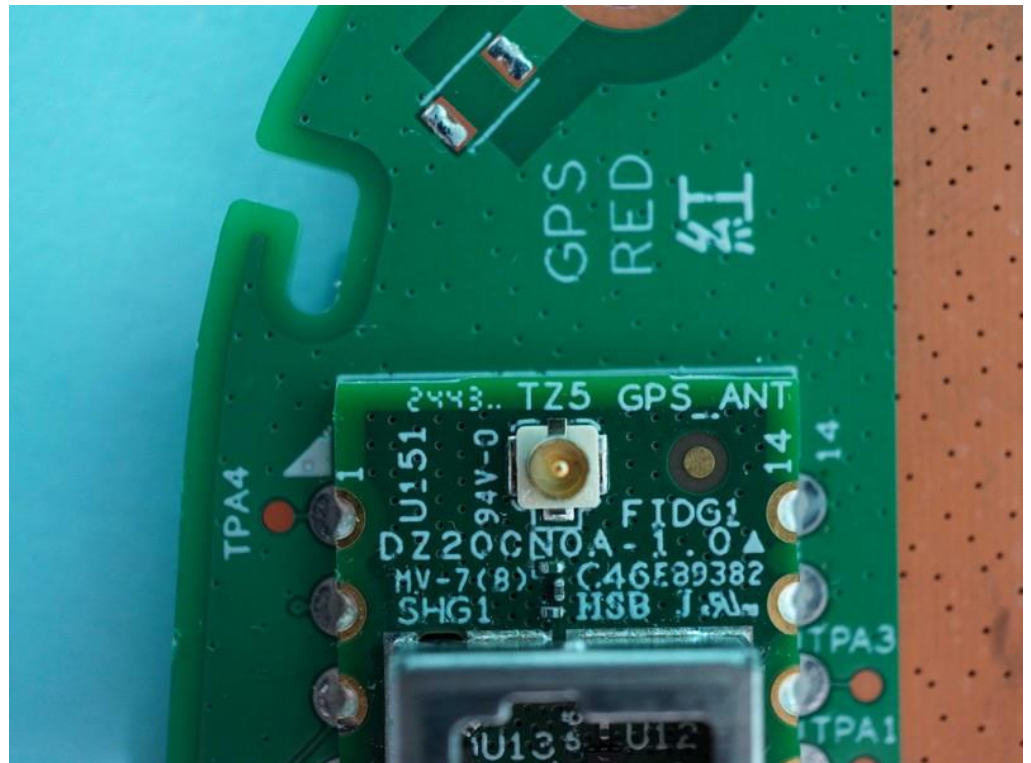
Ant. 1~4
