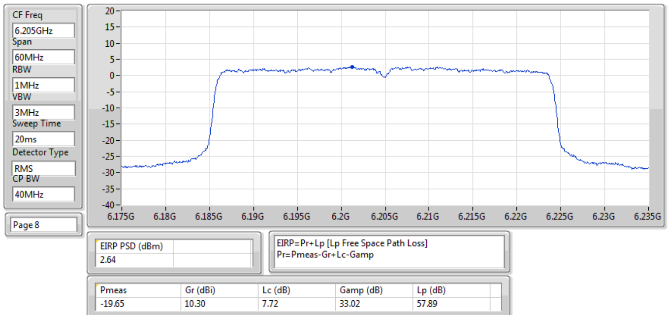
EIRP PSD;Band:6.2G;ax40;BWch:40MHz;Nss:2;(M0);Nant:2;Ch:6205MHz;TX
