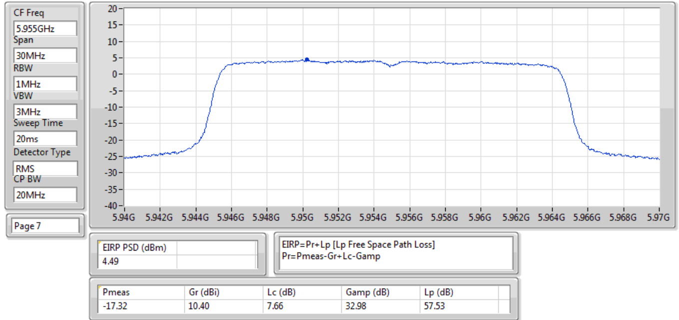
EIRP PSD;Band:6.2G;ax20;BWch:20MHz;Nss:2,(M0);Nant:2;Ch:5955MHz;TX
