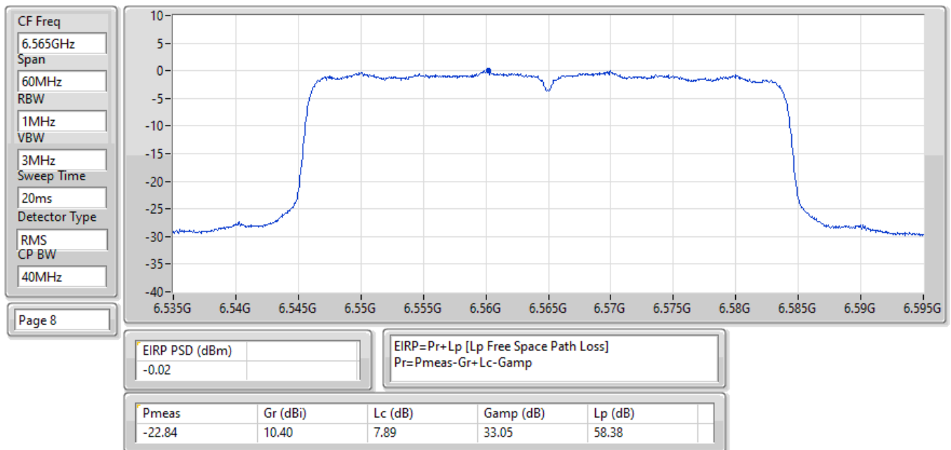
EIRP PSD;Band:6.7G;ax40;BWch:40MHz;Nss:2;(M0);Nant:2;Ch:6565MHz;TX
