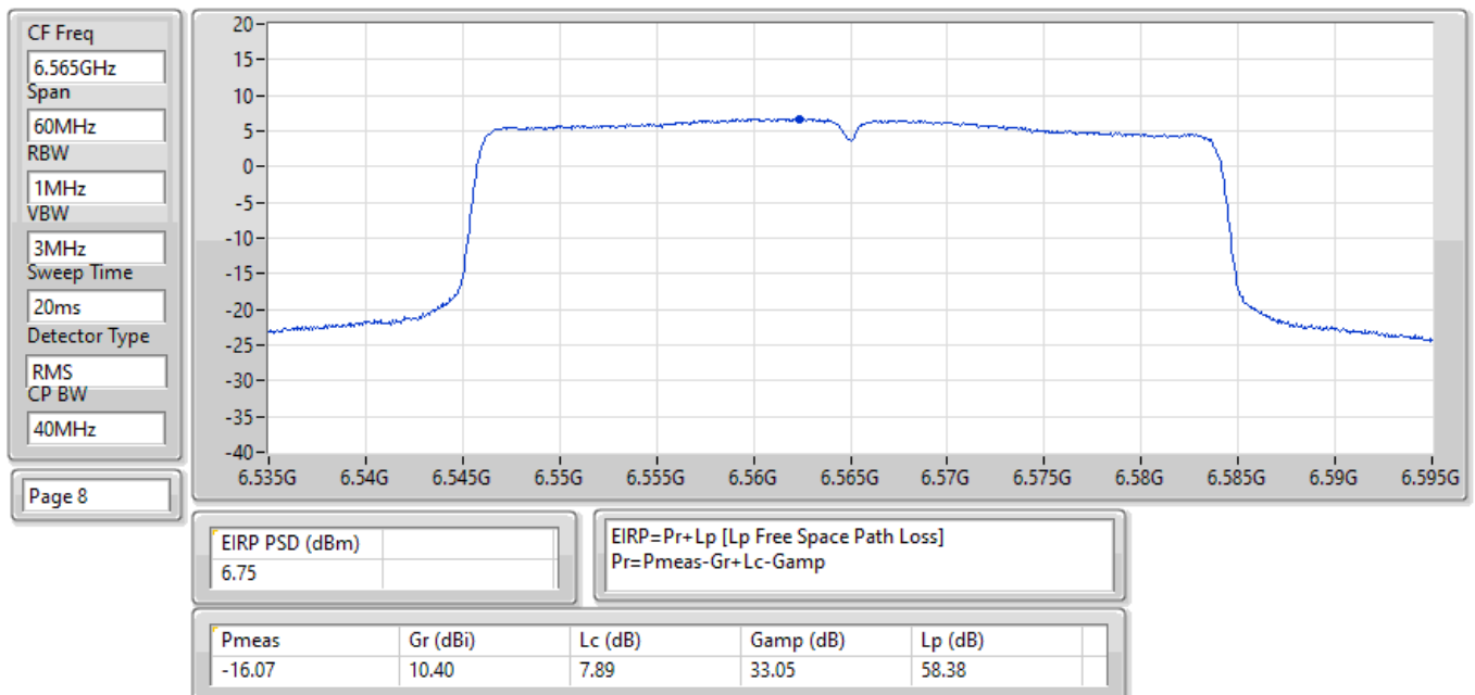
EIRP PSD;Band:6.7G;ax40;BWch:40MHz;Nss:1,(M0);Nant:1;Ch:6565MHz;TX
