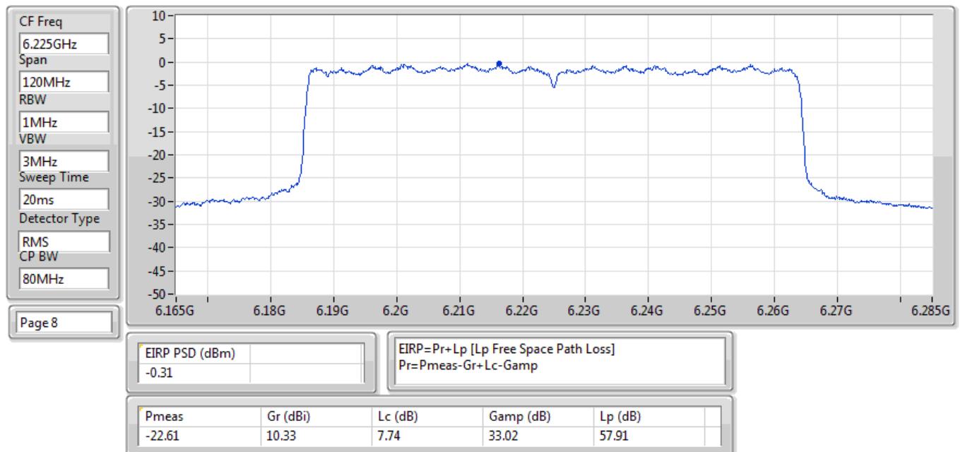
EIRP PSD;Band:6.2G;ax80;BWch:80MHz;Nss:2,(M0);Nant:2;Ch:6225MHz;TX
