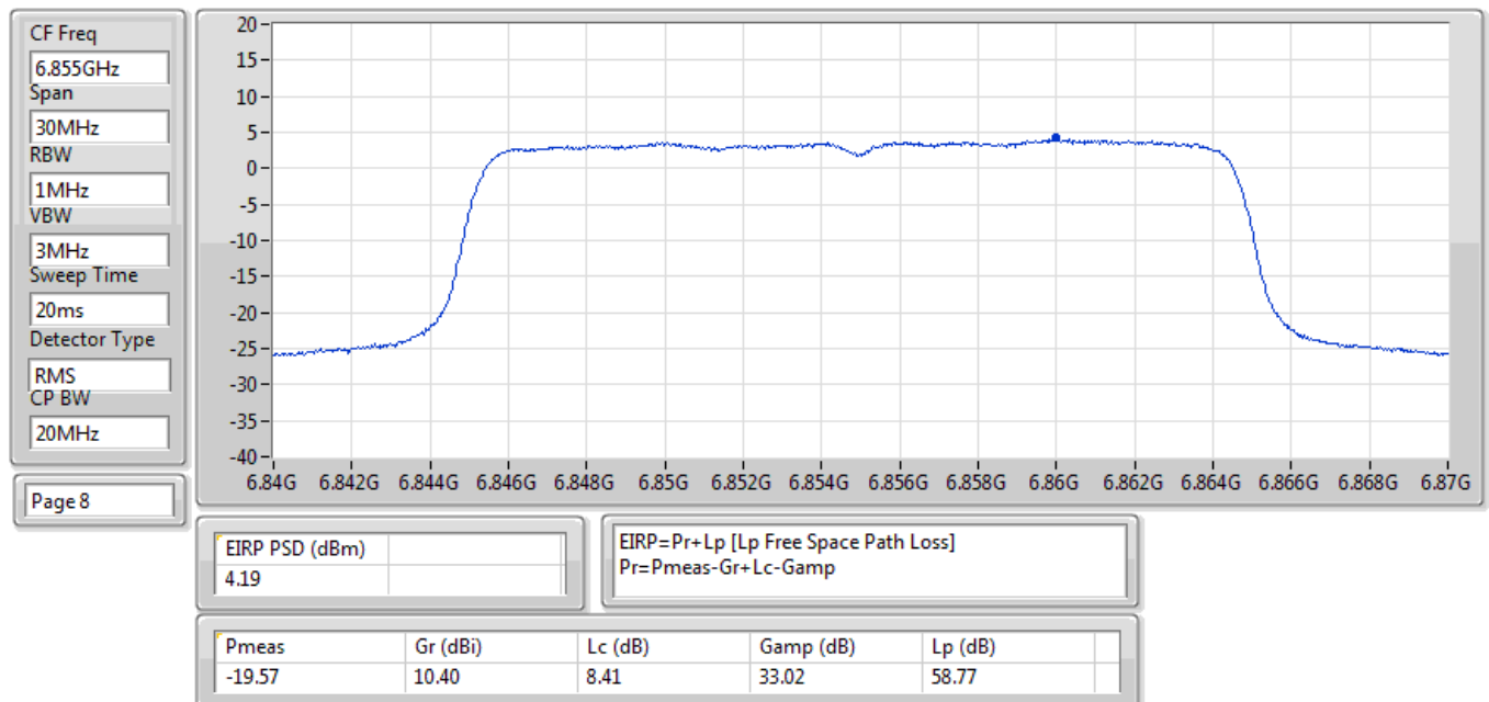
EIRP PSD;Band:6.7G;ax20;BWch:20MHz;Nss:2;(M0);Nant:2;Ch:6855MHz;TX
