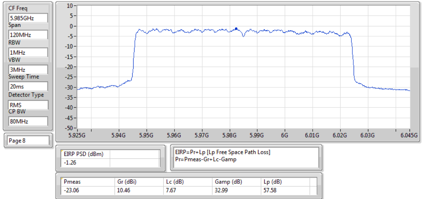
EIRP PSD;Band:6.2G;ax80;BWch:80MHz;Nss:2,(M0);Nant:2;Ch:5985MHz;TX
