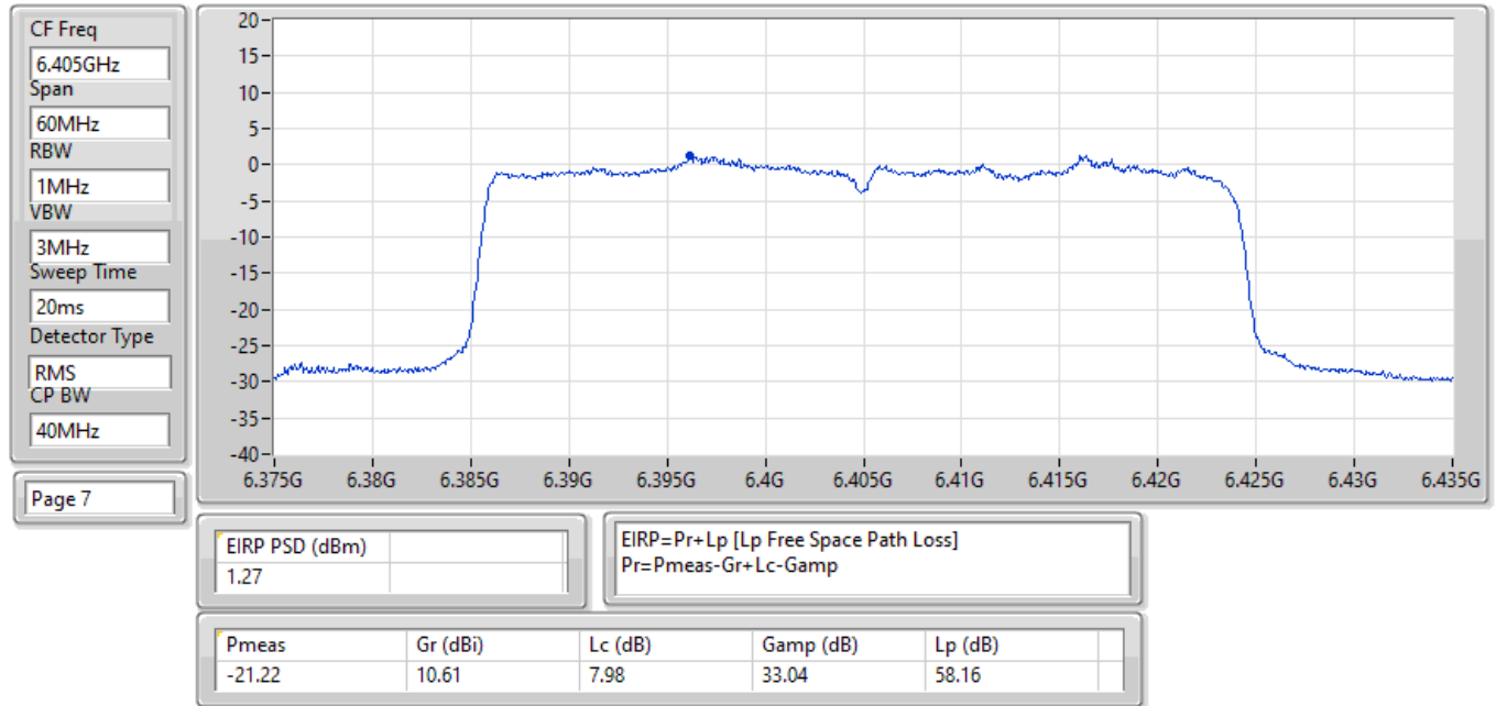
EIRP PSD;Band:6.2G;ax40;BWch:40MHz;Nss:4,(M0);Nant:4;Ch:6405MHz;TX
