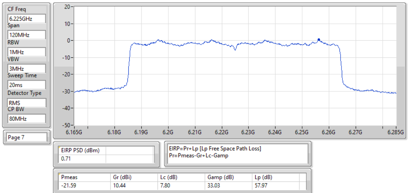
EIRP PSD;Band:6.2G;ax80;BWch:80MHz;Nss:4,(M0);Nant:4;Ch:6225MHz;TX
