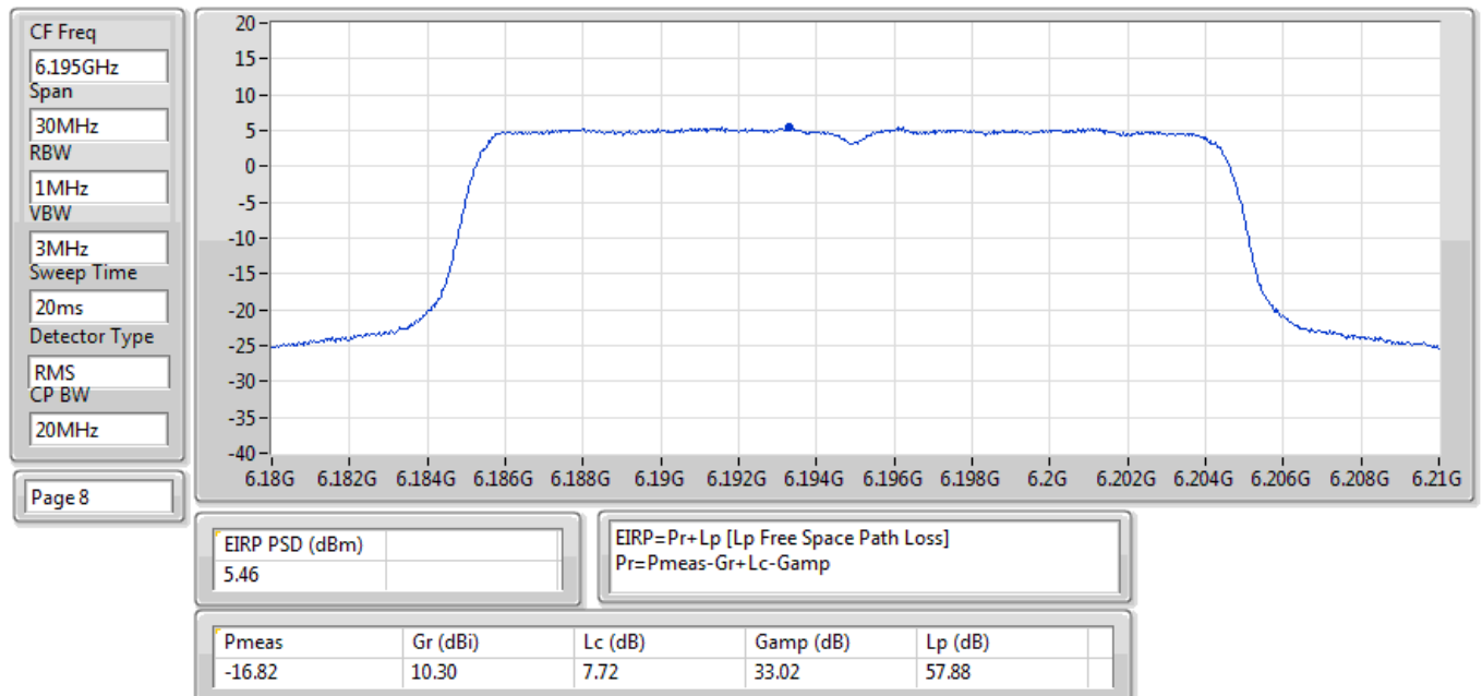
EIRP PSD;Band:6.2G;ax20;BWch:20MHz;Nss:2,(M0);Nant:2;Ch:6195MHz;TX
