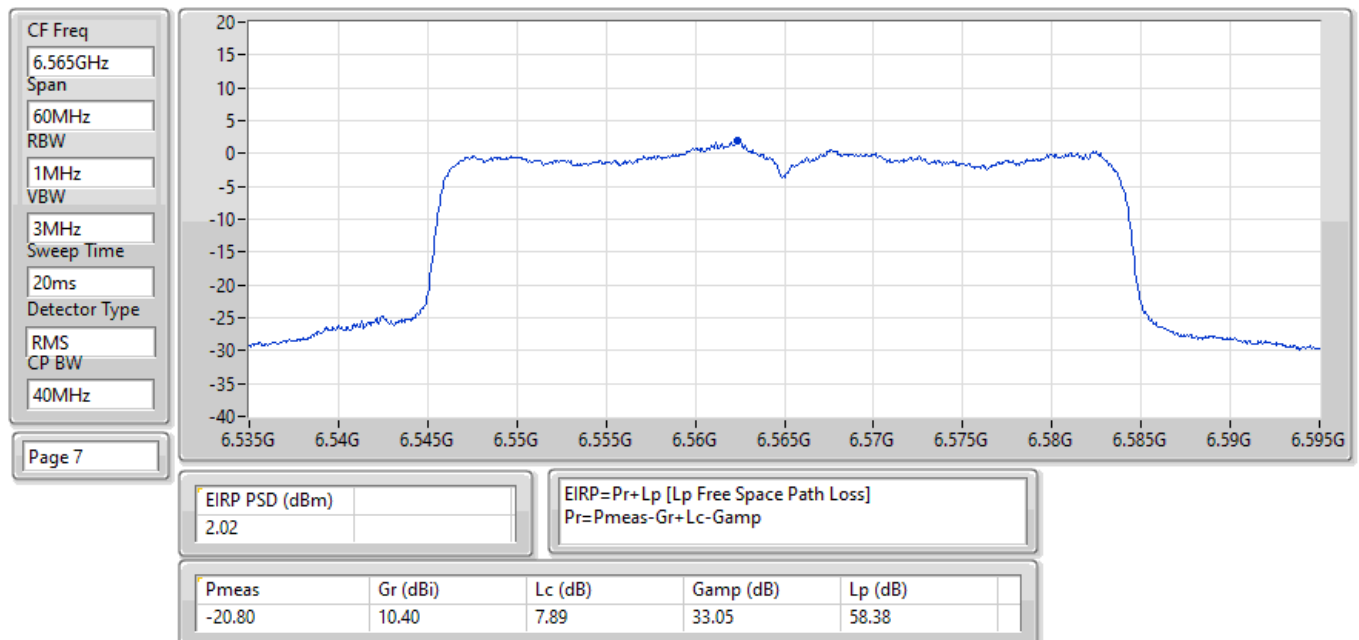
EIRP PSD;Band:6.7G;ax40;BWch:40MHz;Nss:4,(M0);Nant:4;Ch:6565MHz;TX
