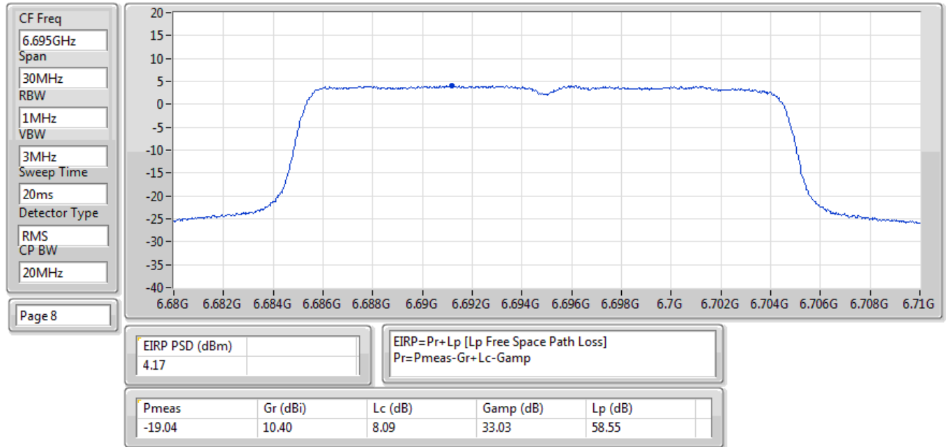
EIRP PSD;Band:6.7G;ax20;BWch:20MHz;Nss:2;(M0);Nant:2;Ch:6695MHz;TX
