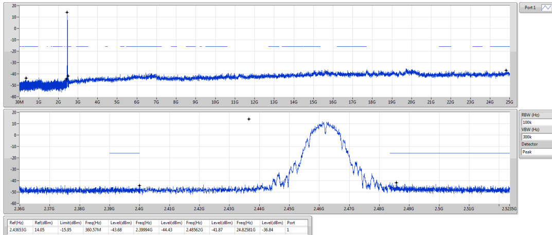
802.11b_Nss1,(1Mbps)_1TX 2462MHz
