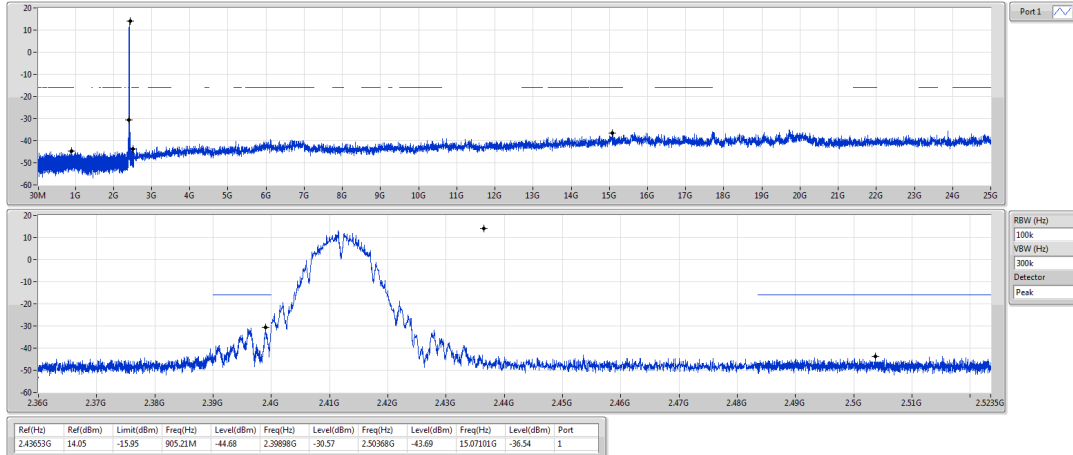
802.11b_Nss1,(1Mbps)_1TX 2412MHz
