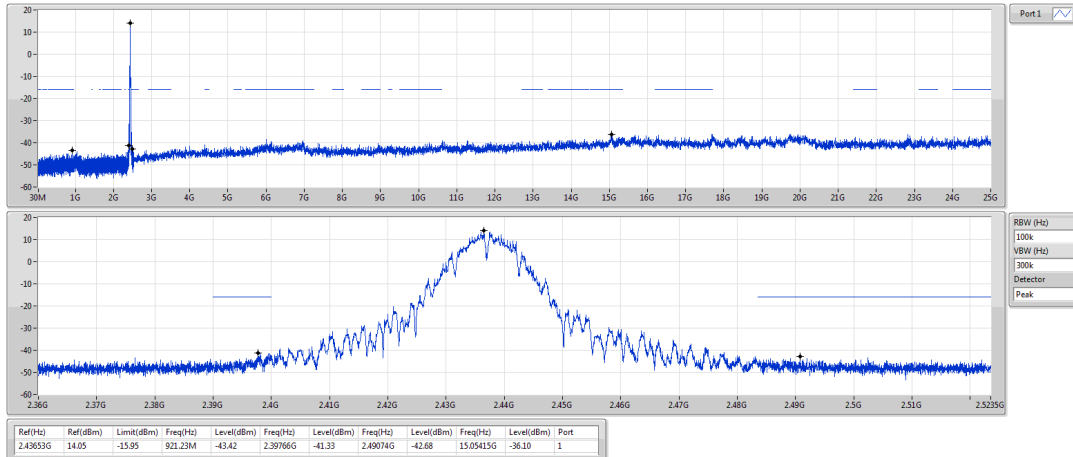
802.11b_Nss1,(1Mbps)_1TX 2437MHz
