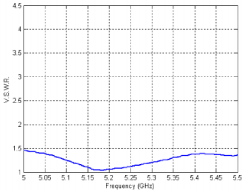
V.S.W.R
