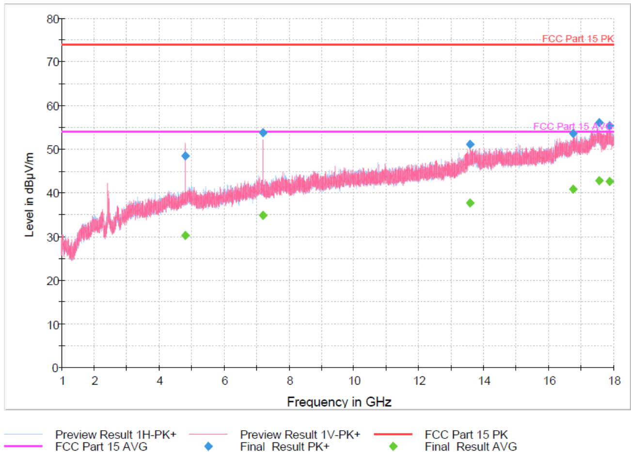
Plot 24. 1-18GHz, BLE-2402MHz
