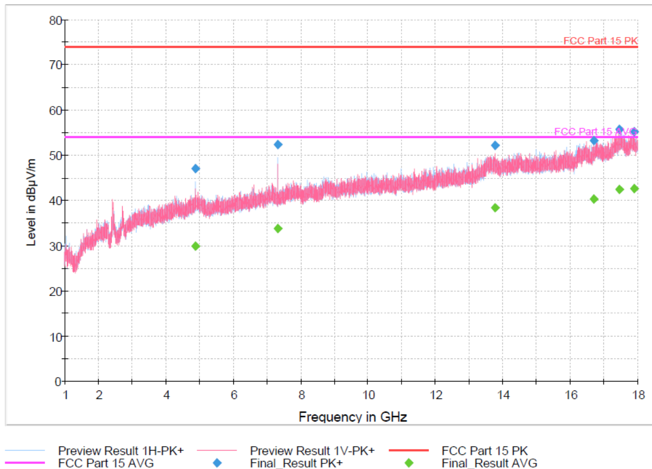
Plot 25. 1-18GHz, BLE-2440MHz
