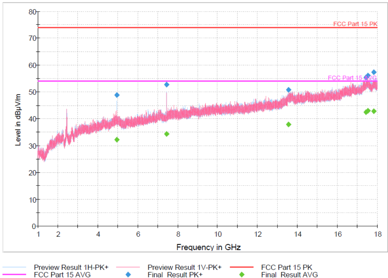
Plot 26. 1-18GHz, BLE-2480MHz
