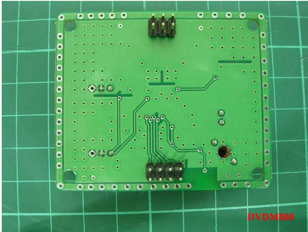
RF module
