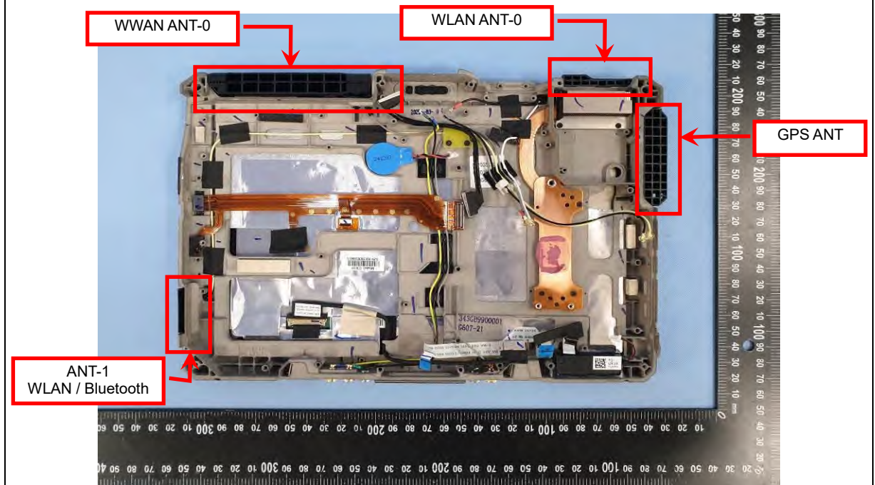
EUT Photo (46)
