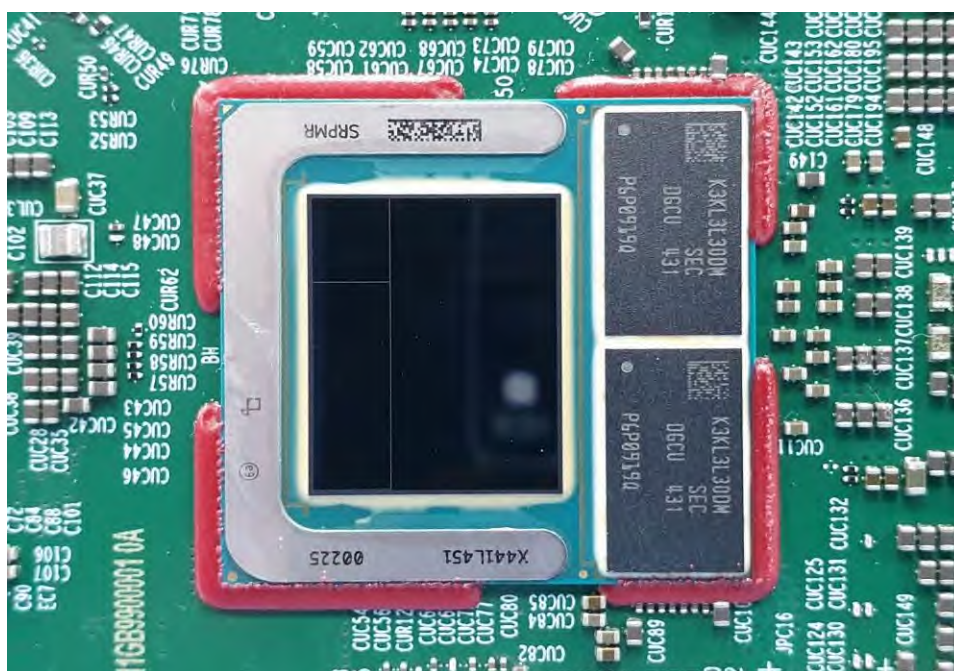
EUT Photo (40)
