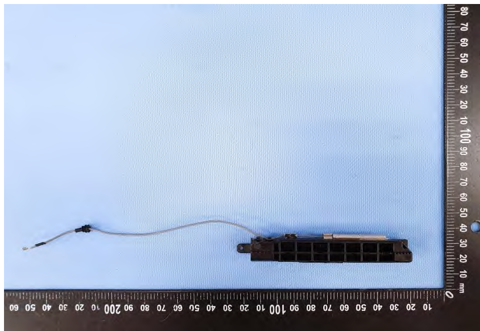
EUT Photo (60)
