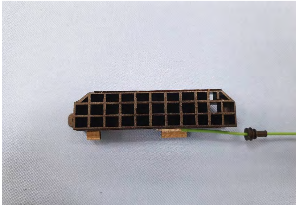
EUT Photo (100)
