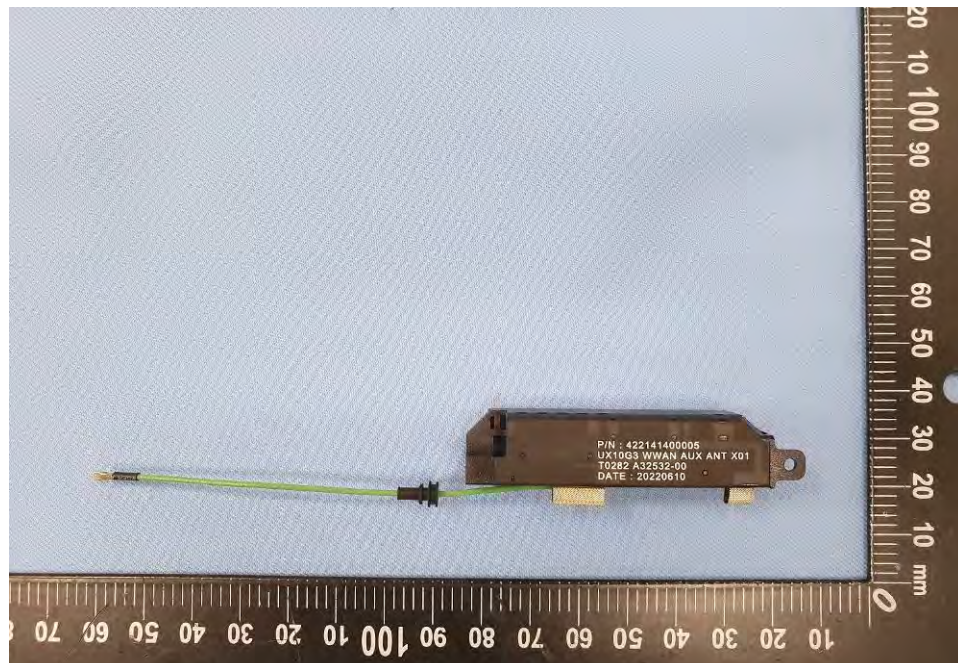
EUT Photo (94)
