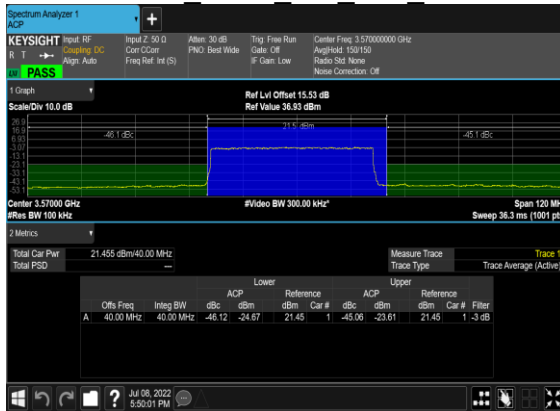
B13_N48(40M)_DFT-s-OFDM_PI_2-BPSK Edge 1RB Right Low CH
