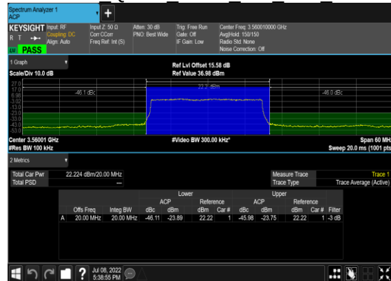
B13_N48(20M)_DFT-s-OFDM QPSK Edge 1RB Right Low CH
