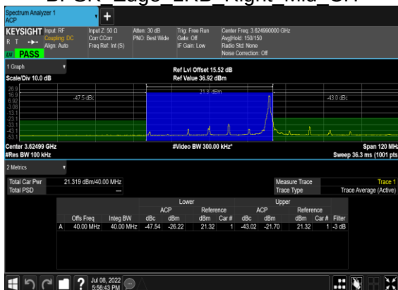
B13_N48(40M)_DFT-s-OFDM_PI_2-BPSK Edge 1RB Right Mid CH
