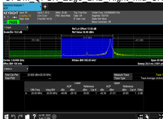
B13_N48(20M)_DFT-s-OFDM QPSK Edge 1RB Right Mid CH
