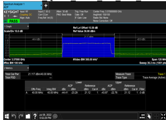
B13_N48(40M)_DFT-s-OFDM QPSK Edge 1RB Right Low CH
