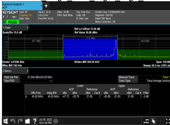
B13_N48(40M)_DFT-s-OFDM_PI_2-BPSK Edge 1RB Right High CH
