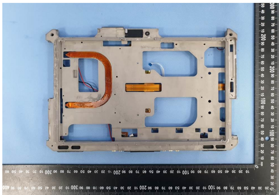
EUT Photo (100)
