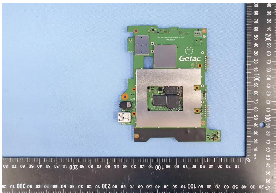
EUT Photo (58)
