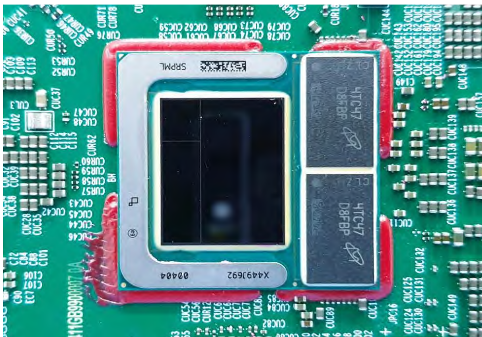
EUT Photo (41)
