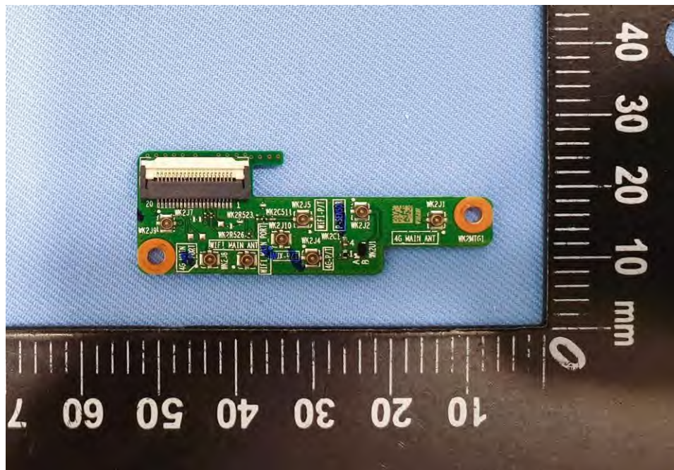
EUT Photo (19)
