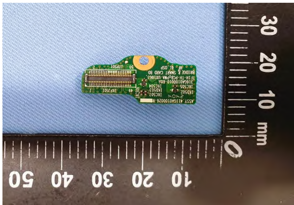
EUT Photo (37)
