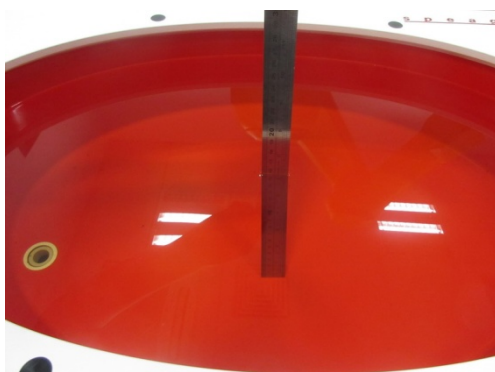
HSL(1750-2600MHz)
