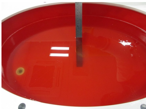
HSL(1750-2600MHz)
