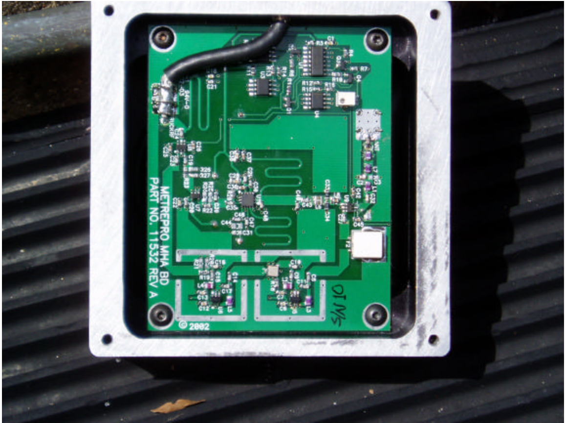
MHA PCB Top
