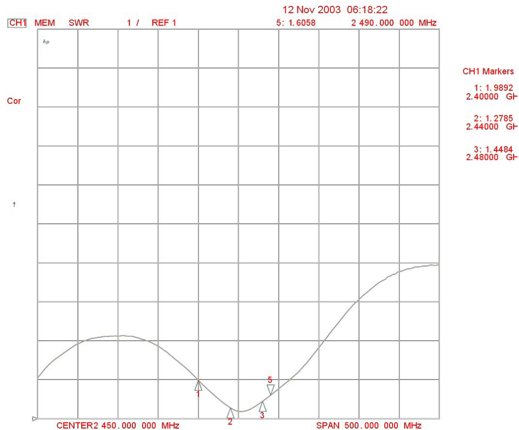
Fig 2. VSWR
