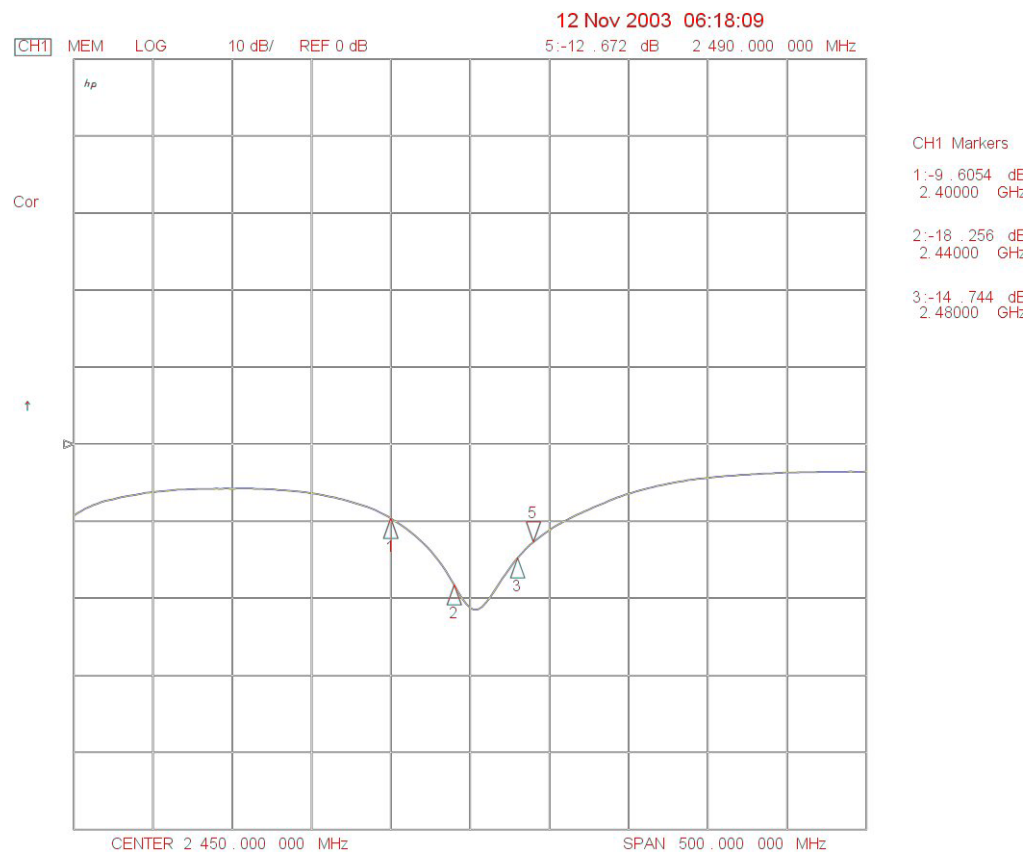
Fig 2. VSWR
