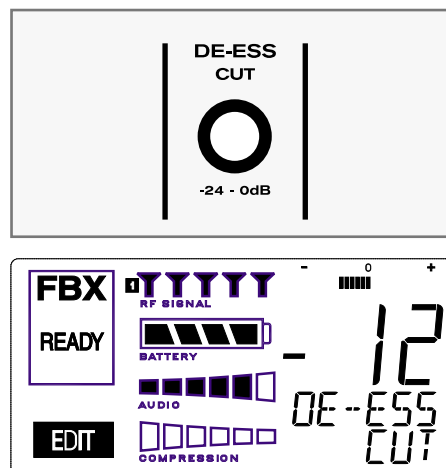
Fig. 9a: De-esser
