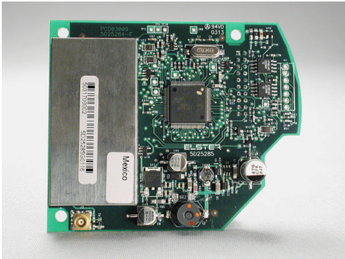
LAN Board
