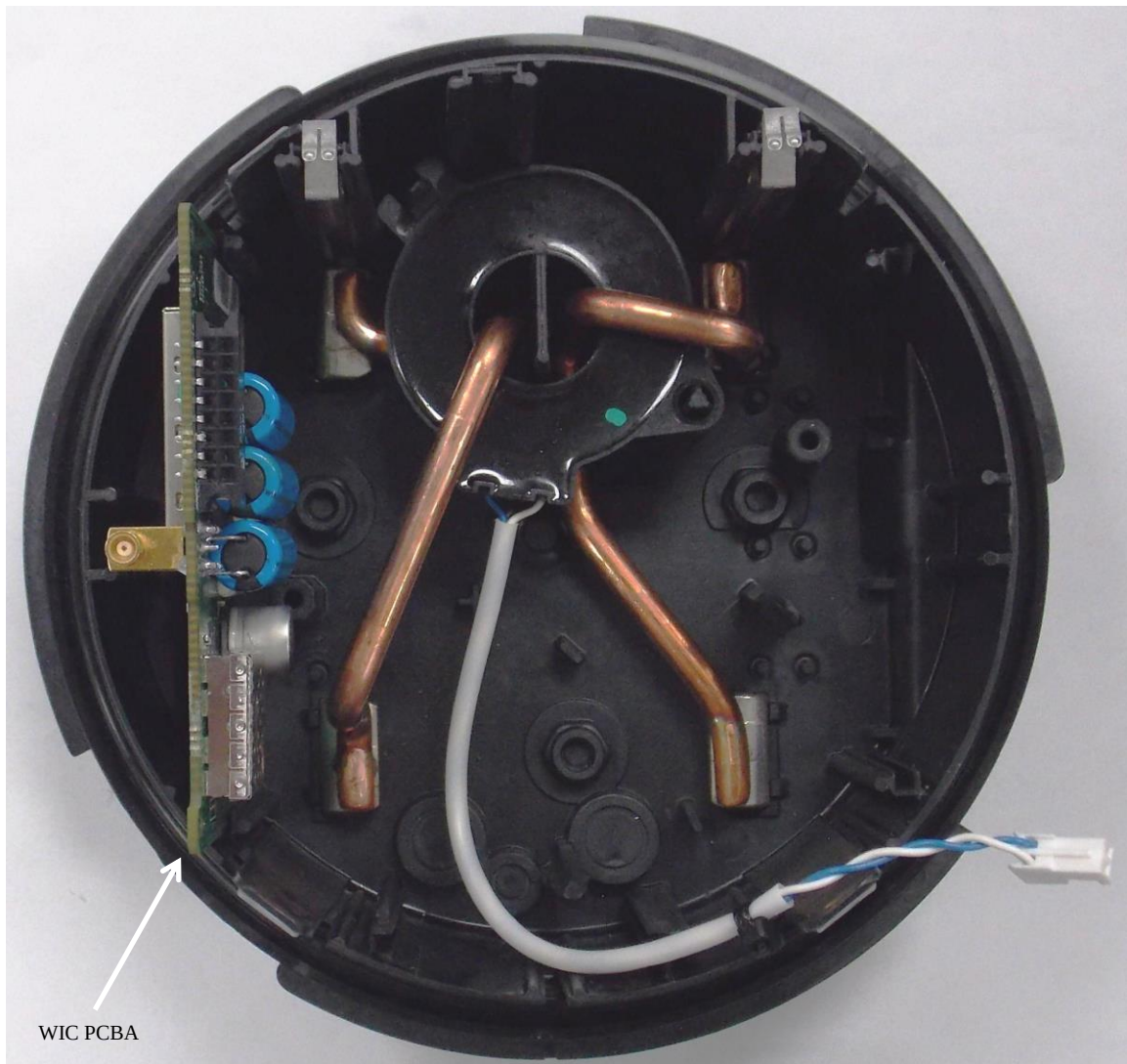
REXUniversal ® Form 2S meter base & WIC PCBA (Model # RXUEVV)
