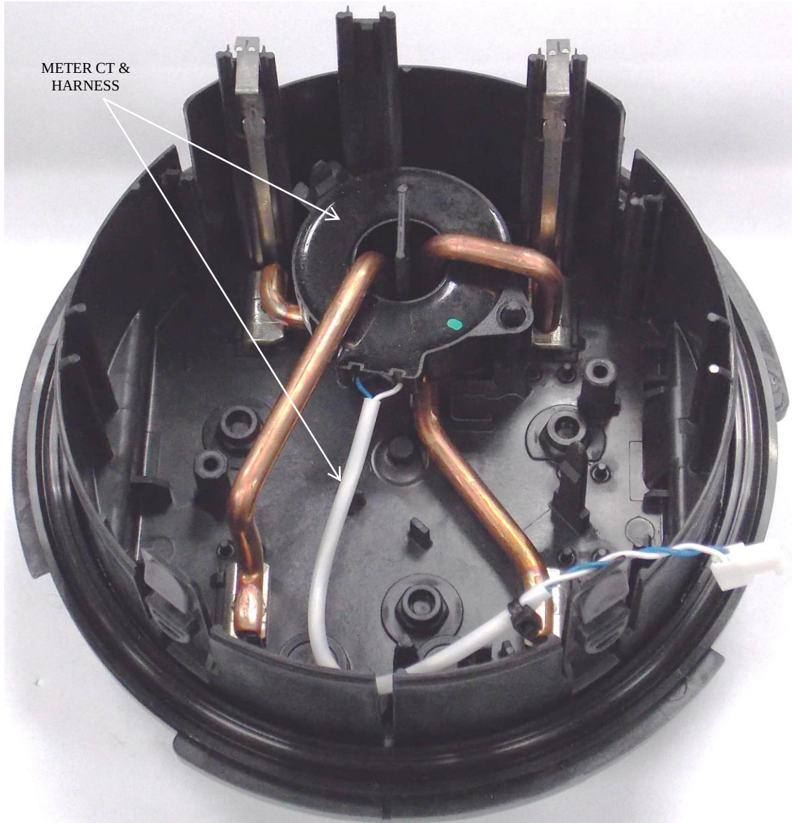
REXUniversal® Form 2S meter base (Model # RXUEVV)
