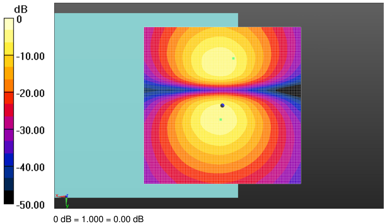
Fig B.5 T-Coil WCDMA 850
