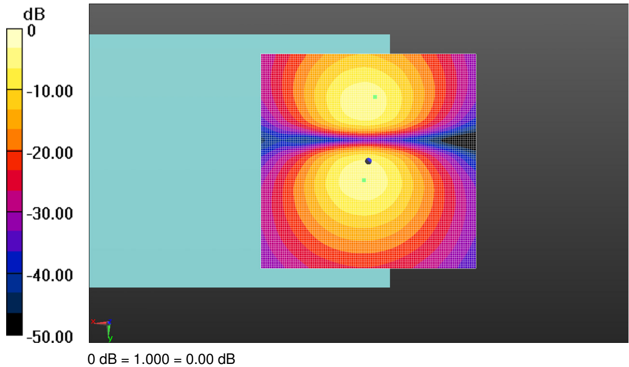
Fig B.9 T-Coil WCDMA 1900
