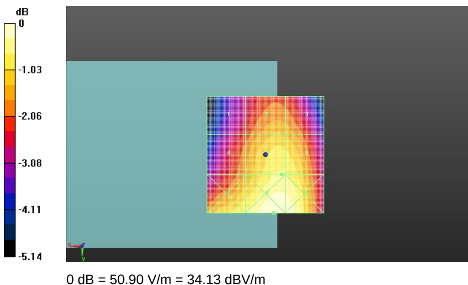
Fig A.3 HAC RF E-Field GSM 850 Low
