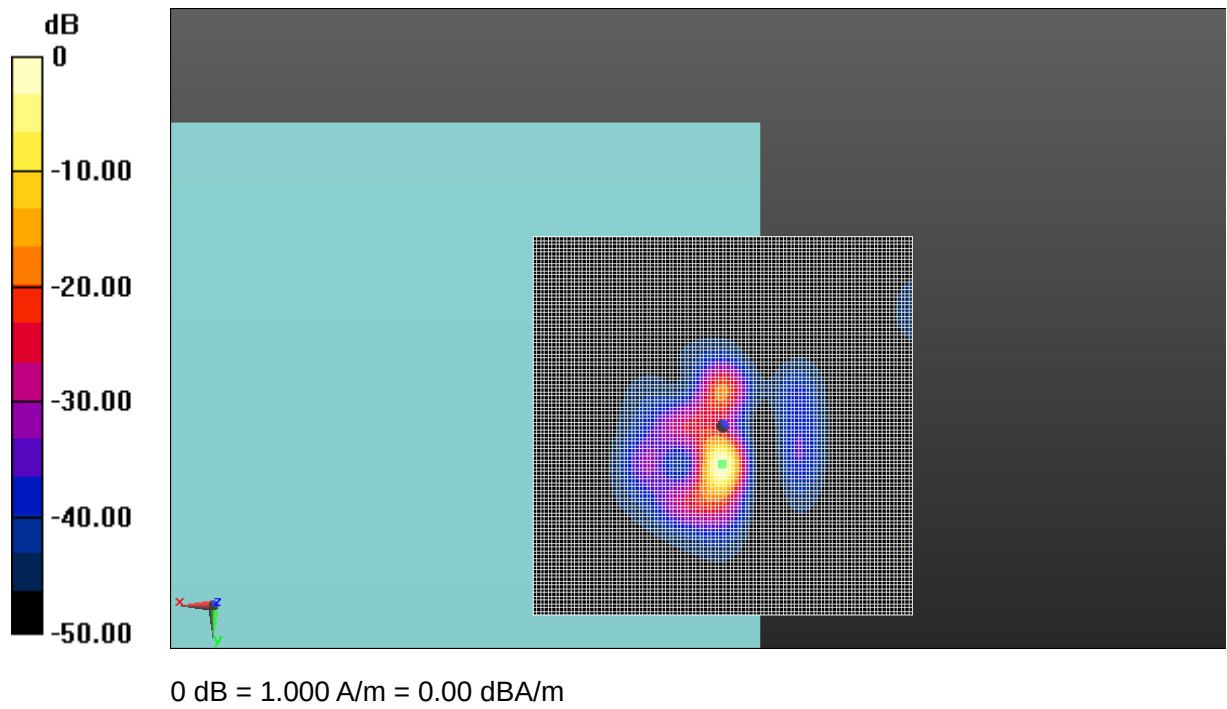
Fig A.35 T-Coil EDGE 850
