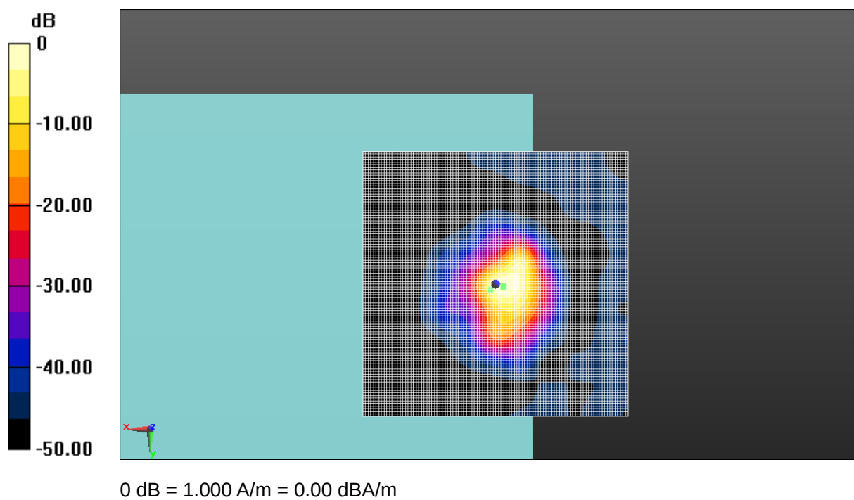
Fig A.39 T-Coil WCDMA B2
