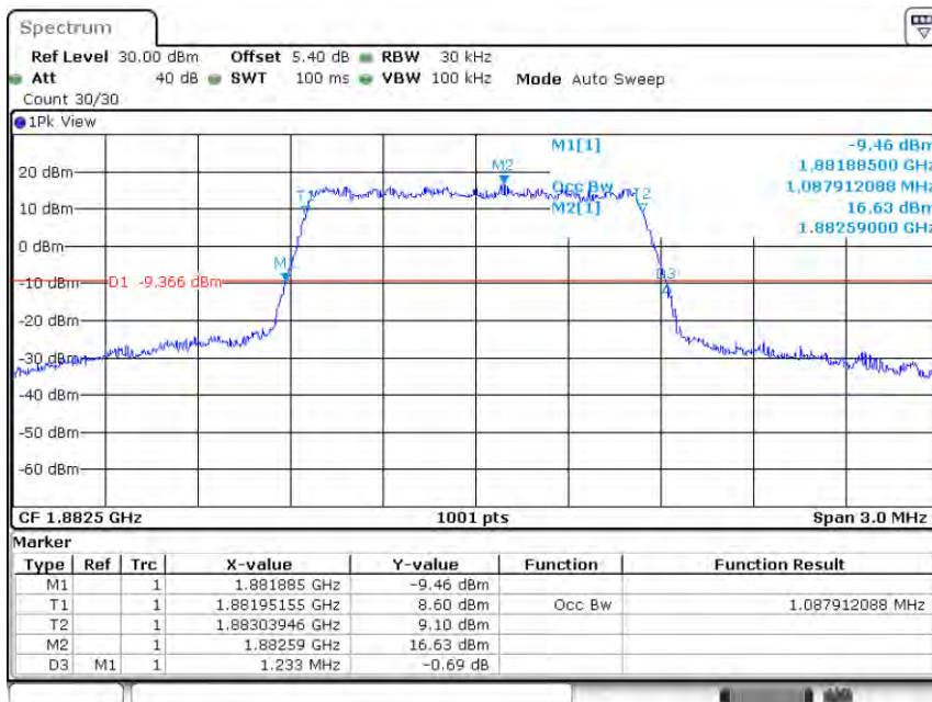
Band25-1.4MHz-QPSK-26365-6RB#0-1.088
