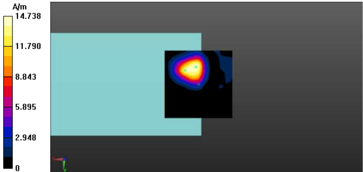
Fig A.31 T-Coil WCDMA B4-Z
