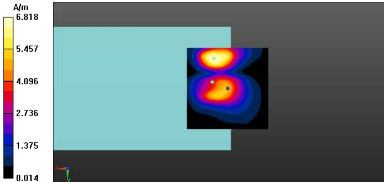
Fig A.31 T-Coil WCDMA B4-Y
