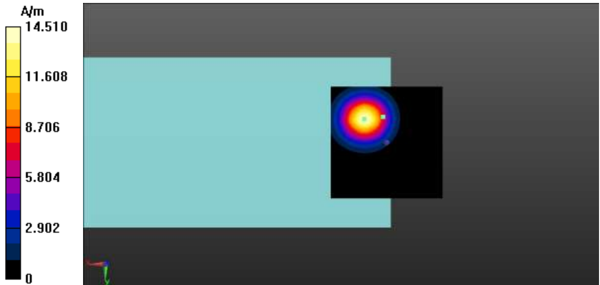
Fig A.6 T-Coil WCDMA B2-Z
