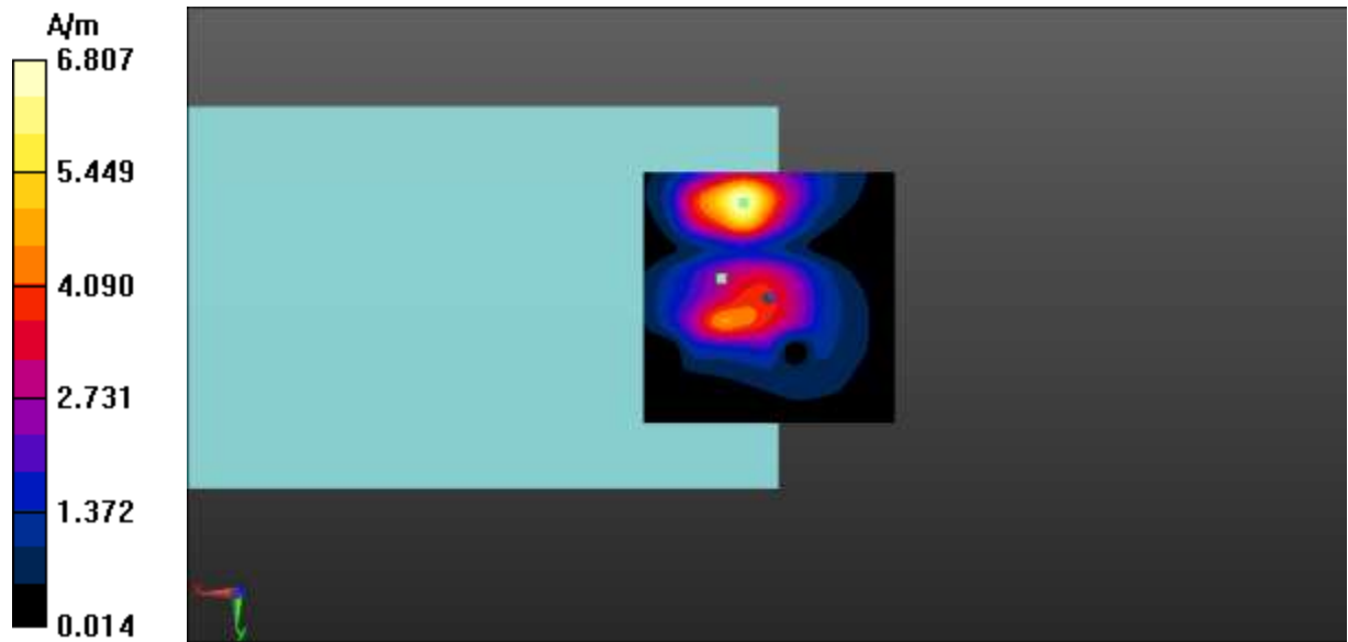
Fig A.30 T-Coil WCDMA B2-Y
