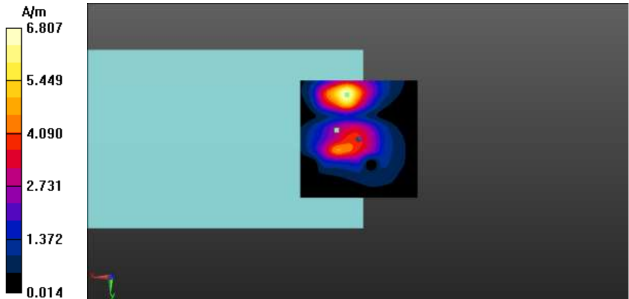
Fig A.6 T-Coil WCDMA B2-Y
