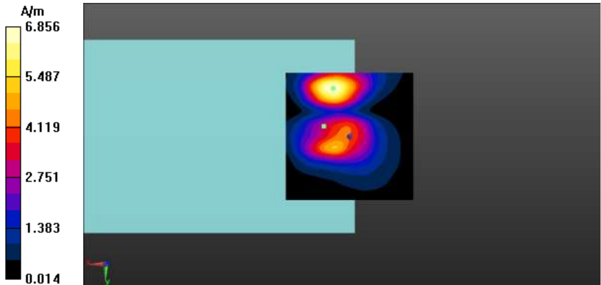
Fig A.8 T-Coil WCDMA B5-Y
