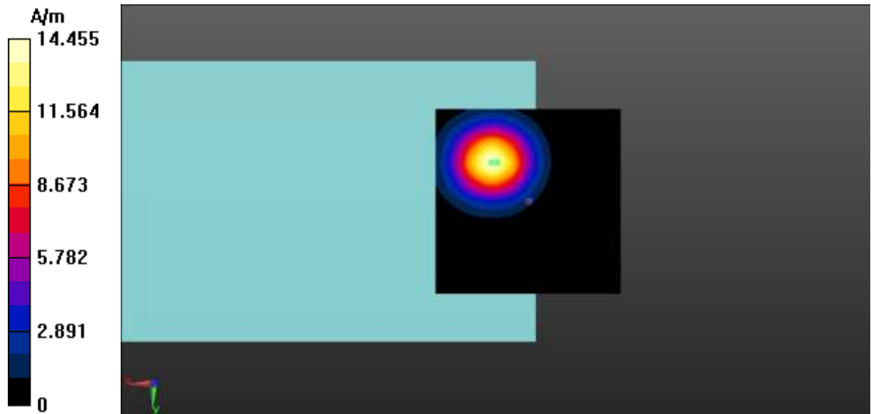
Fig A.25 T-Coil GSM 850-Z
