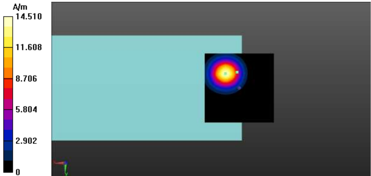
Fig A.30 T-Coil WCDMA B2-Z
