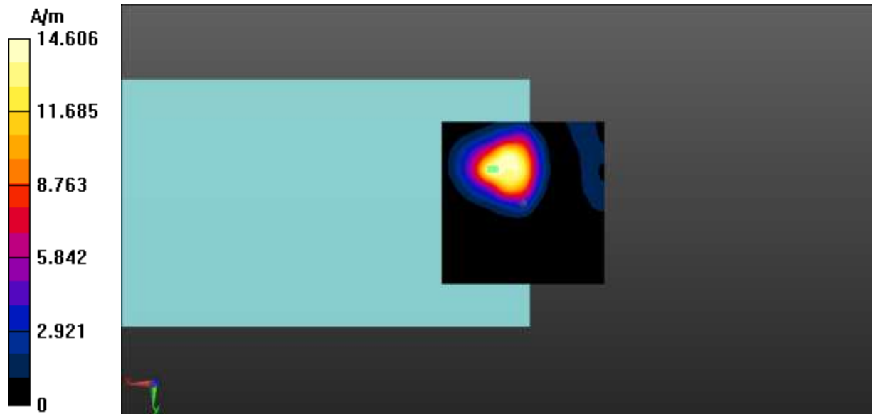
Fig A.32 T-Coil WCDMA B5-Z
