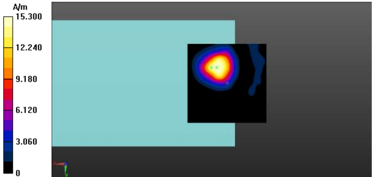
Fig A.5 T-Coil CDMA BC10-Z
