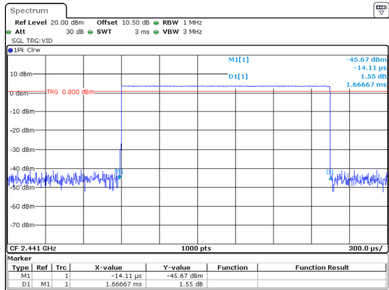
DH3_Hop_2441 1.667ms
