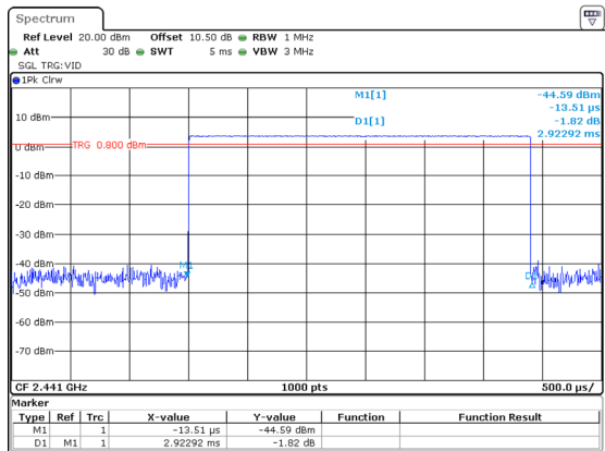
DH5_Hop_2441 2.923ms
