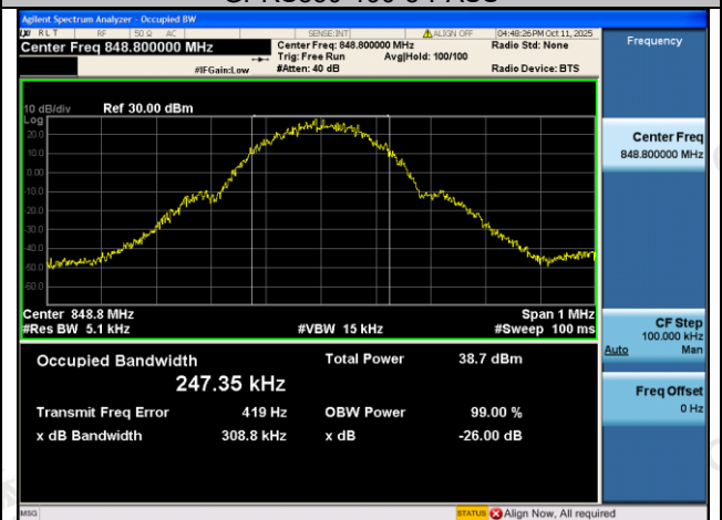
GPRS850-251-5-PASS
