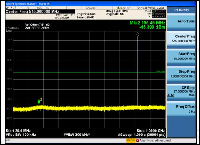
GPRS850-128-5-30~1000MHz-PASS
