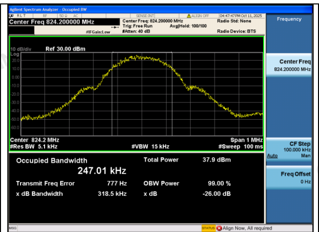
GPRS850-128-5-PASS
