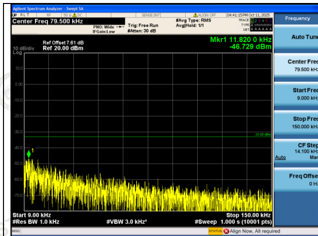
GSM850-128-5-0.009~0.15MHz-PASS
