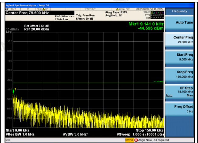
GPRS850-128-5-0.009~0.15MHz-PASS
