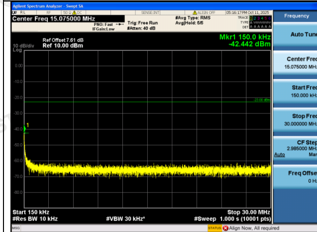
GSM850-251-5-0.15~30MHz-PASS
