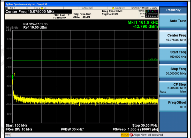
GPRS850-128-5-0.15~30MHz-PASS
