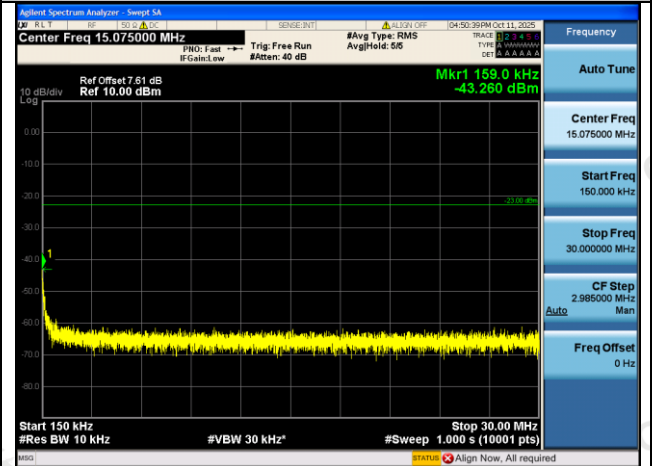
GPRS850-251-5-0.15~30MHz-PASS
