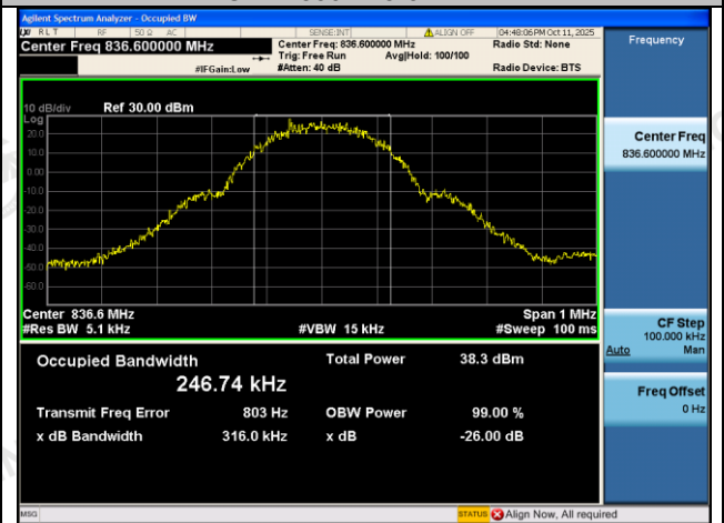
GPRS850-190-5-PASS
