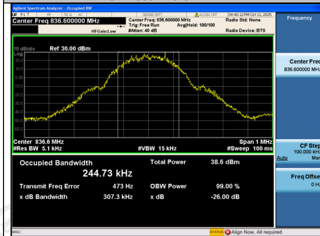
GSM850-190-5-PASS
